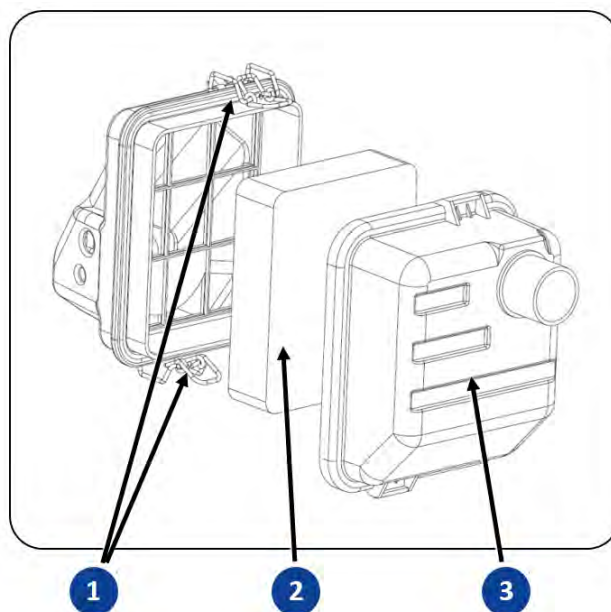
Abb. 9-6 Luftfiltereinsatz ausbauen
