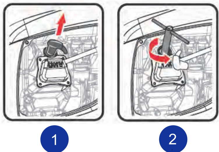
Abb. 9-7 Zündkerze ausbauen
