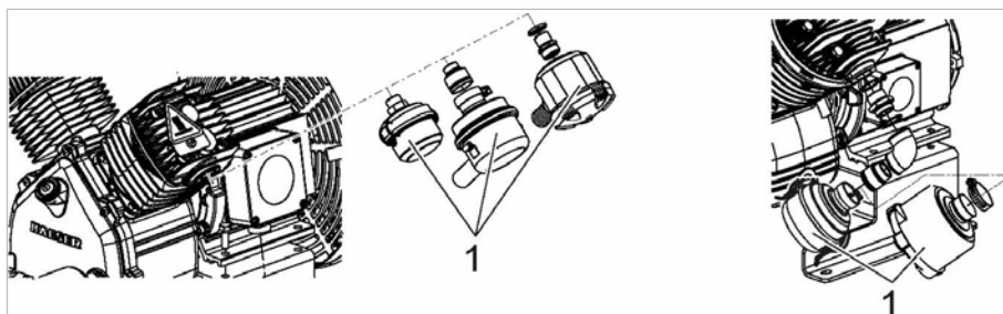
Abb. 7 Luftfilter montieren
