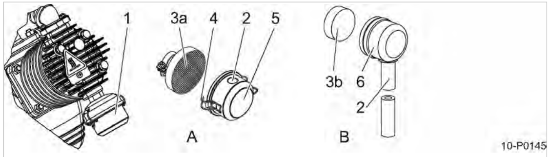
Abb. 13 Luftfilter warten
