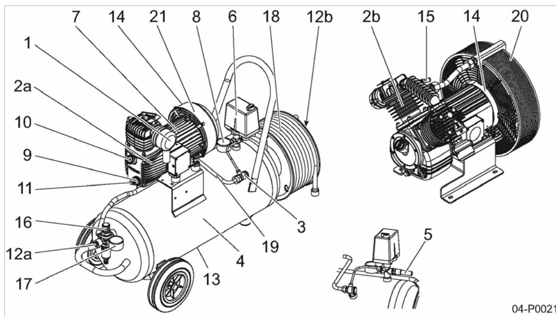
Abb. 2 Übersicht Maschine
