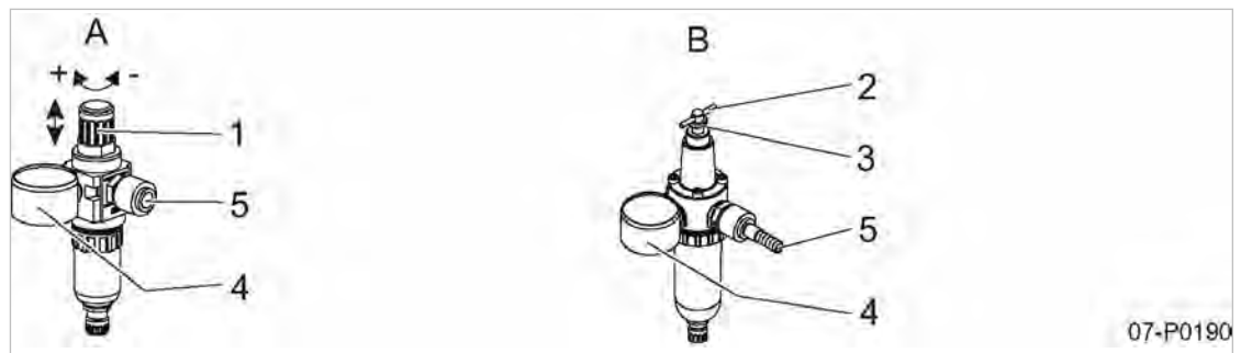
Abb. 10 Filterdruckminderer einstellen
