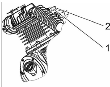
Abb. 19 Sicherheitsventil am Sammelrohr prüfen
