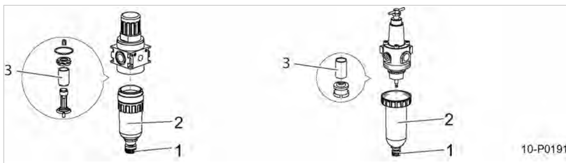
Abb. 25 Filterdruckminderer reinigen
