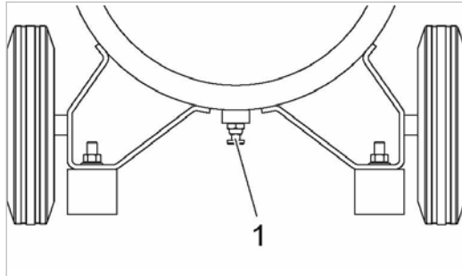
Abb. 21 Kondensat ablassen
