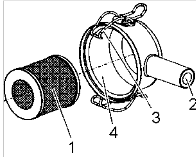
Abb. 14 Option H9: Luftfilter (geräuschkämpfend) warten
