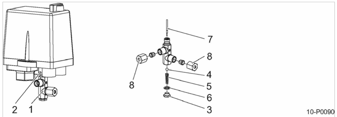
Abb. 24 Entlastungsventil am Druckschalter warten
