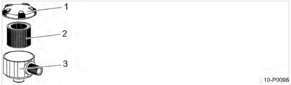
Abb. 15 Option H10: Luftfilter (mit Kunststoffgehäuse) warten
