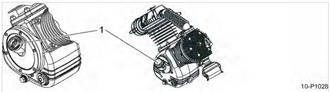
Abb. 17 Kompressoröl nachfüllen
