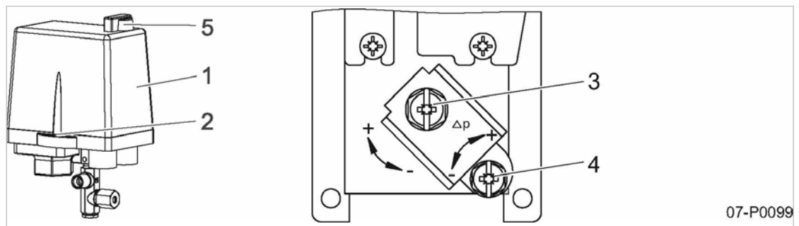
Abb. 9 Netzdruck einstellen
