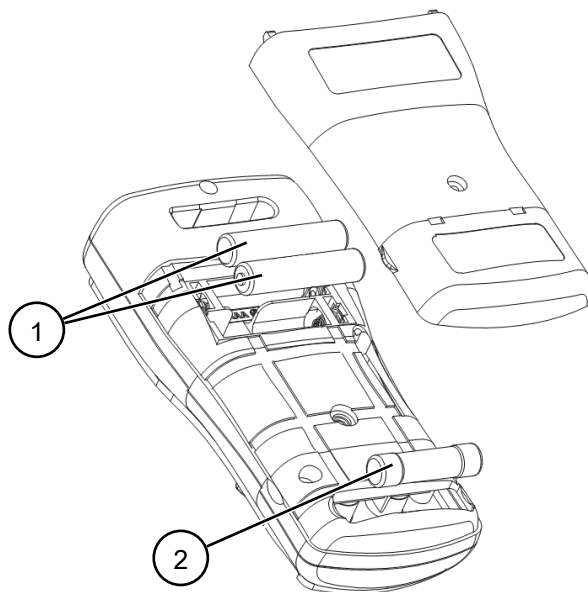
Abb. 16: Batteriewechsel (beispielhaft)
