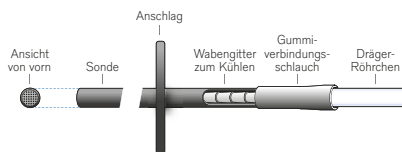
Schema der Heißluftsonde
