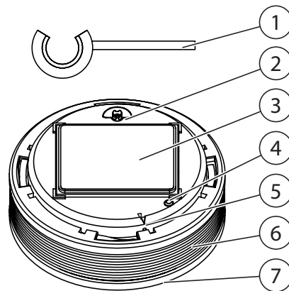
Abb. 1 Bedienelemente
