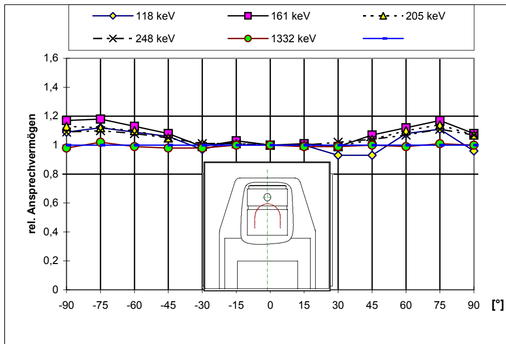
Diagramm 3b Richtungsabhängigkeit des Ansprechvermögens für verschiedene Photonenenergien bezogen auf Haupteinfallrichtung 0 Grad
