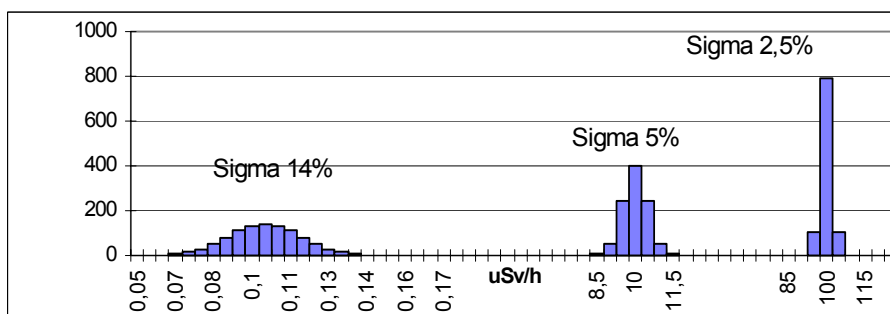
Diagramm 6b Häufigkeitsverteilung von 1000 Messwertablesungen bei Dosisleistungen von 0,1 µSv/h, 10 µSv/h und 100 µSv/h
