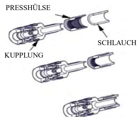
Abbildung 3-2 Austausch der Luftschlauch-Schnellkupplung
