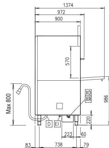
Seitenansicht
