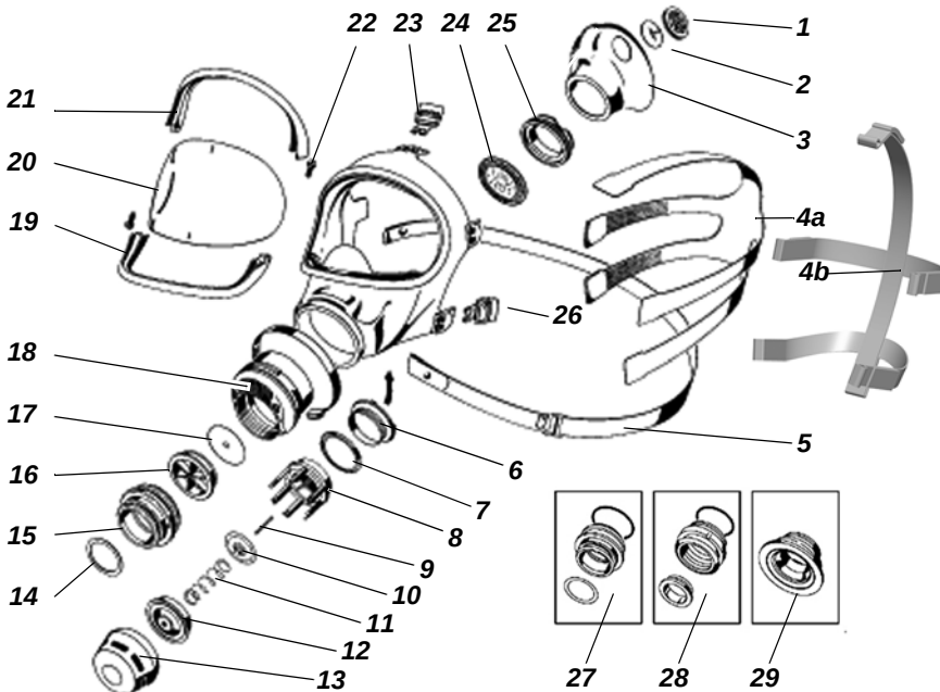
Abb. 4 Vollmaske, Explosionsdarstellung
