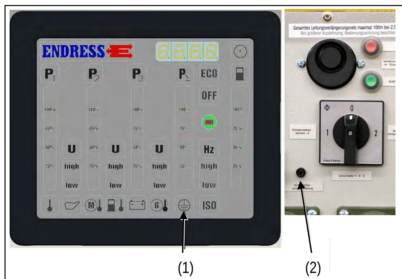
Abb. 4-4: Schutzleiter prüfen
