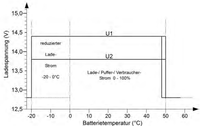
Ladeprogramm „LiFePO4“ 14,4 V, IU1oU2
