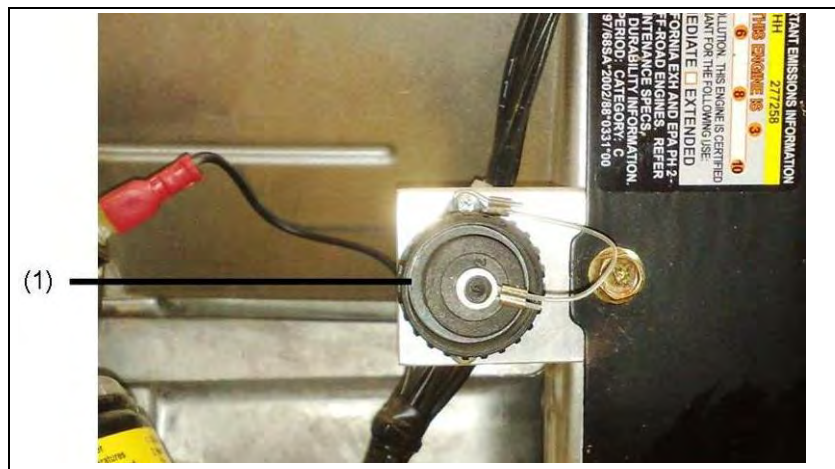
Abb. 5-4: Fernstarteinrichtung anschließen
