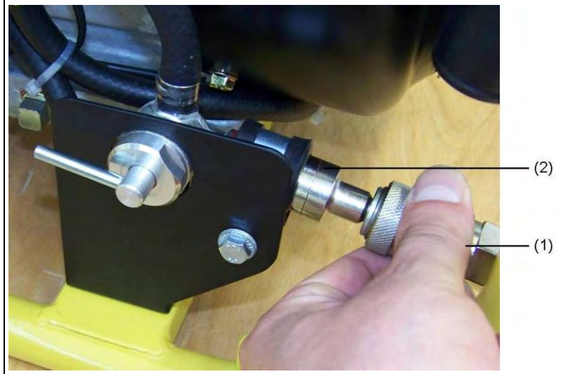
Abb. 5-12: Betankungsgerät anschließen
