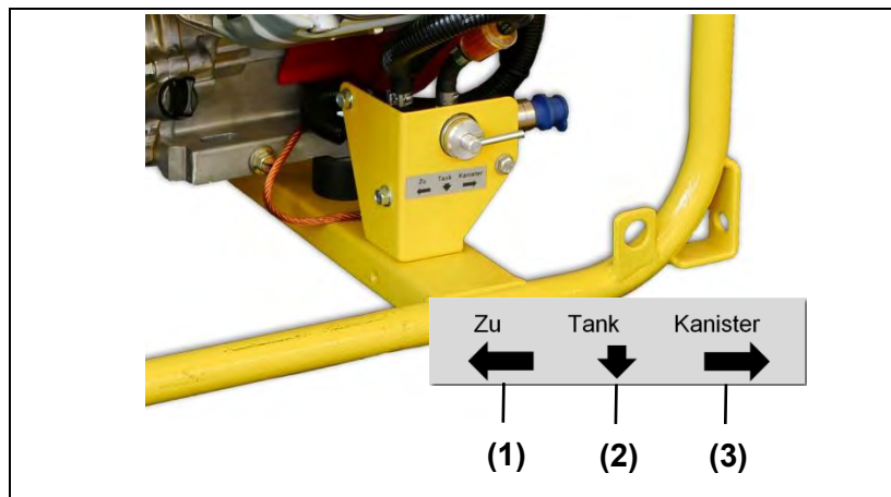
Abb. 5-11: 3 Wege Kraftstoffhahn
