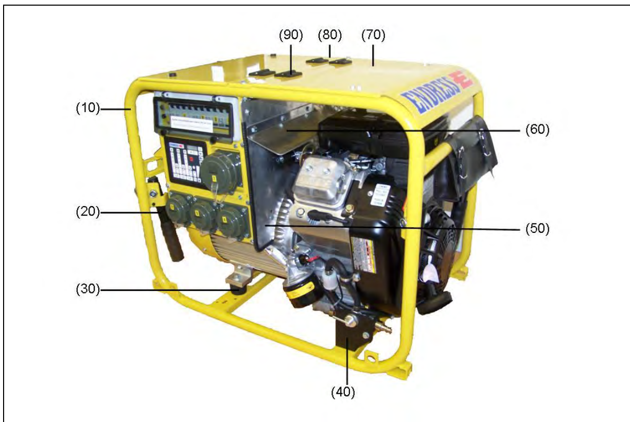
Abb. 9-1: Ersatzteile der Bedien- und Generatorseite
