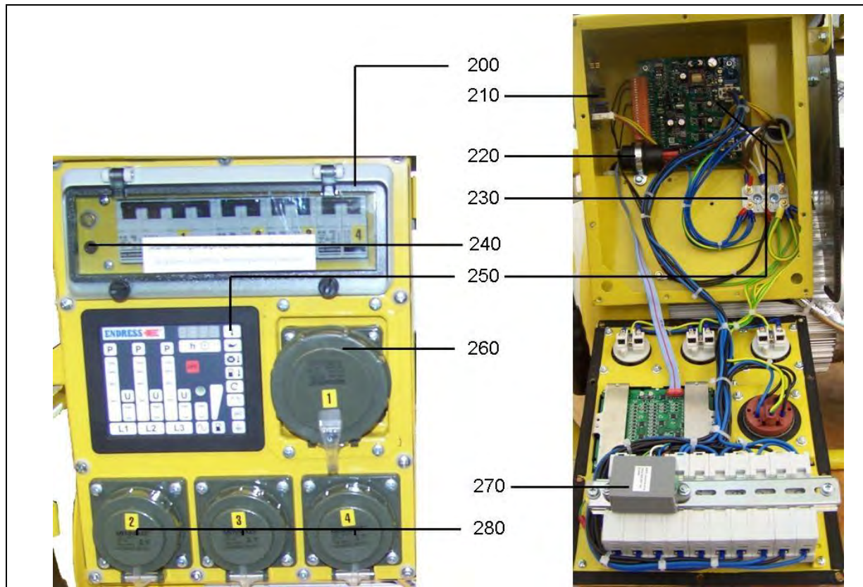
Abb. 9-3: Ersatzteile Generator und Elektronik
