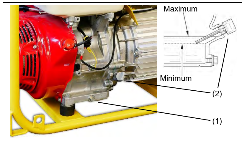
Abb. 6-2: Ölmesstab
