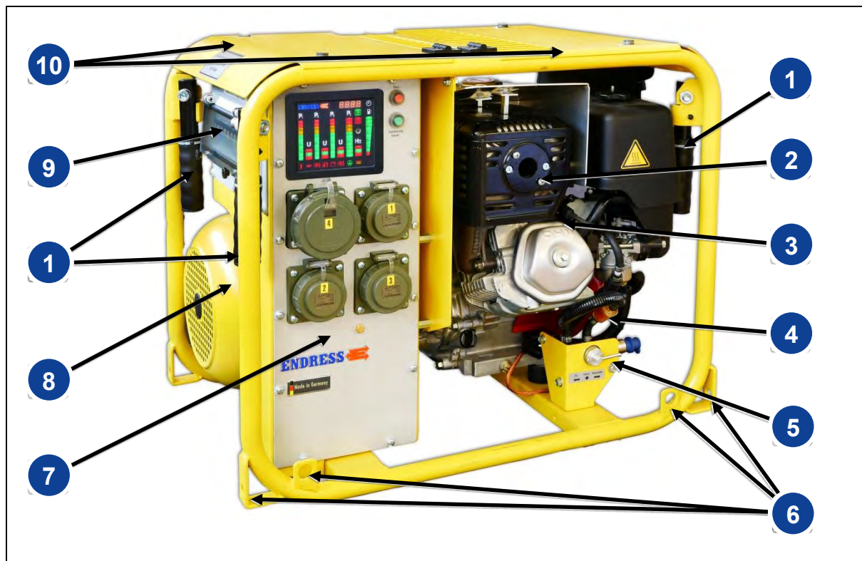
Abb. 3-2: Bestandteile der Bedien- und Generatorseite
