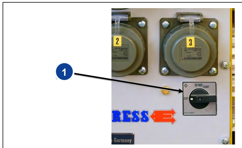
Abb. 4-3: Elektrostart
