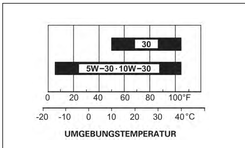
Abb. 6-1: Viskositätsbereiche Motoröl
