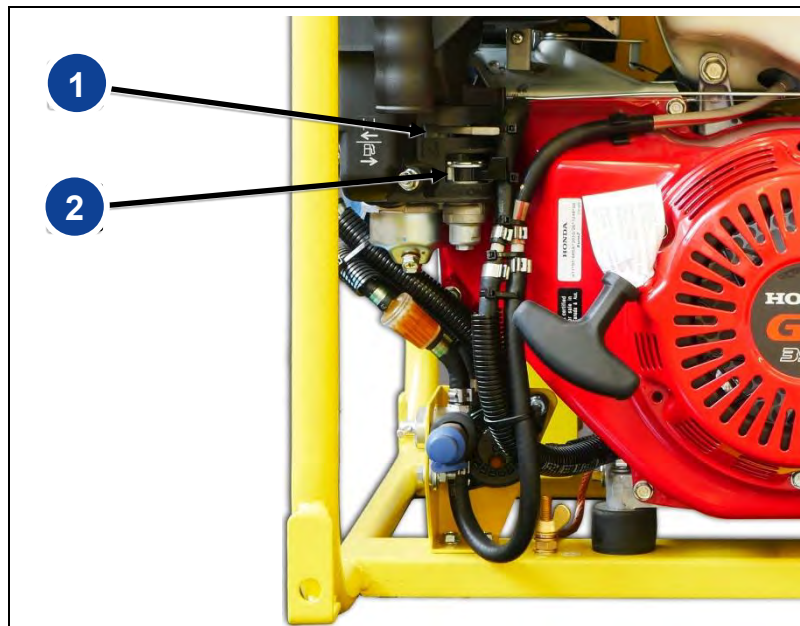
Abb. 4-1: Hebel Kraftstoffhahn und Choke
