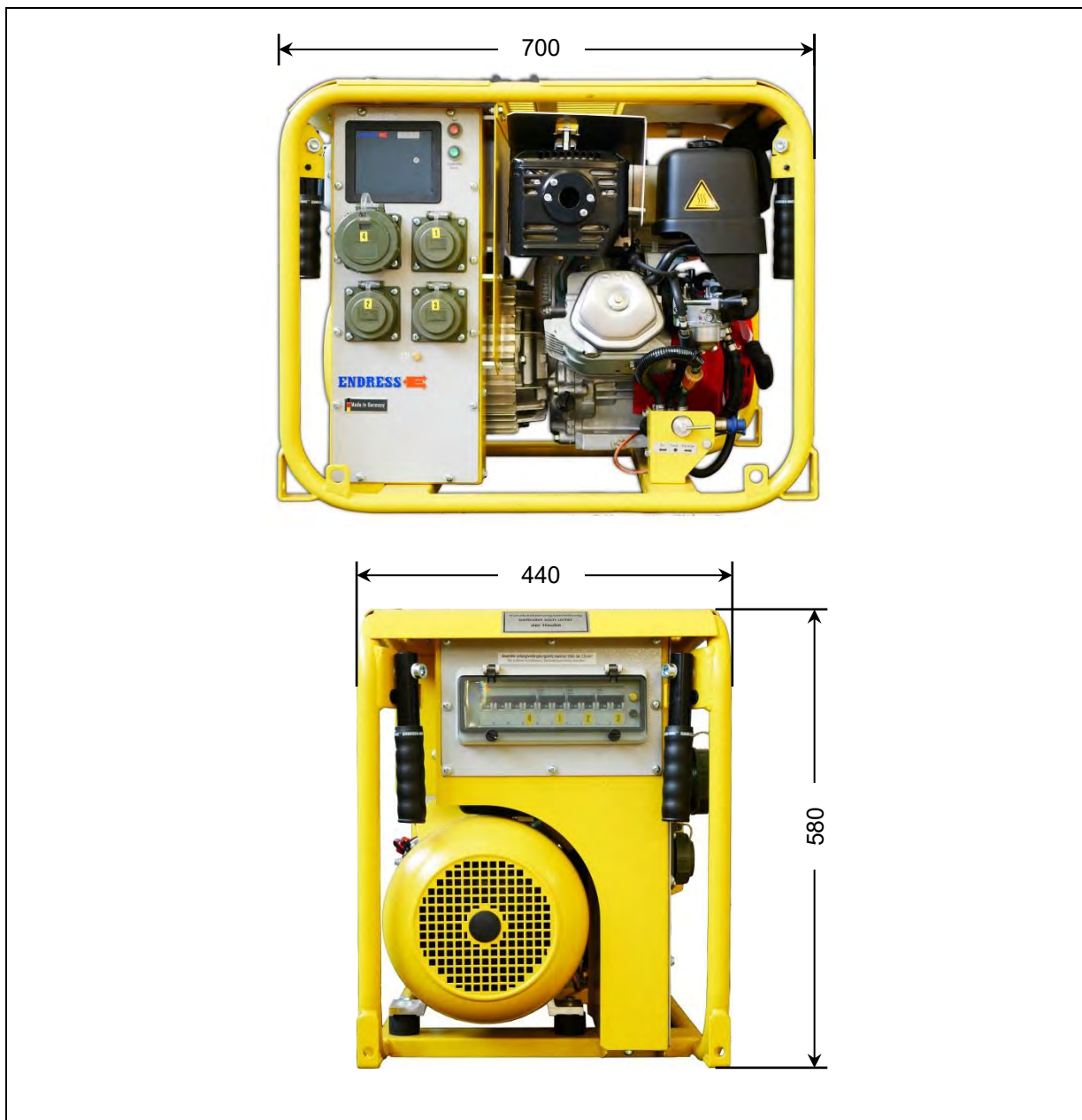
Abb. 8-1: Maße des Stromerzeugers
