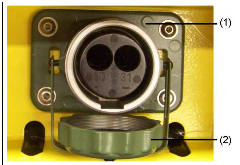
Abb. 5-6: Fremdstartereinrichtung anschließen
