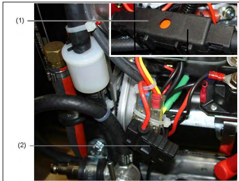
Abb. 6-4: Sicherung tauschen
