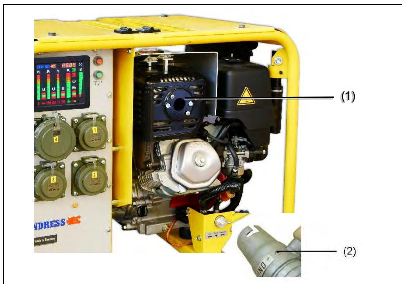
Abb. 5-13 Abgasschlauch anschließen
