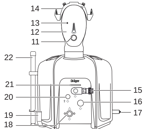
Dräger Quaestor 8000 (Ansicht von vorn)
