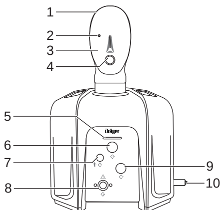
Dräger Quaestor 6000 (Ansicht von vorn)
