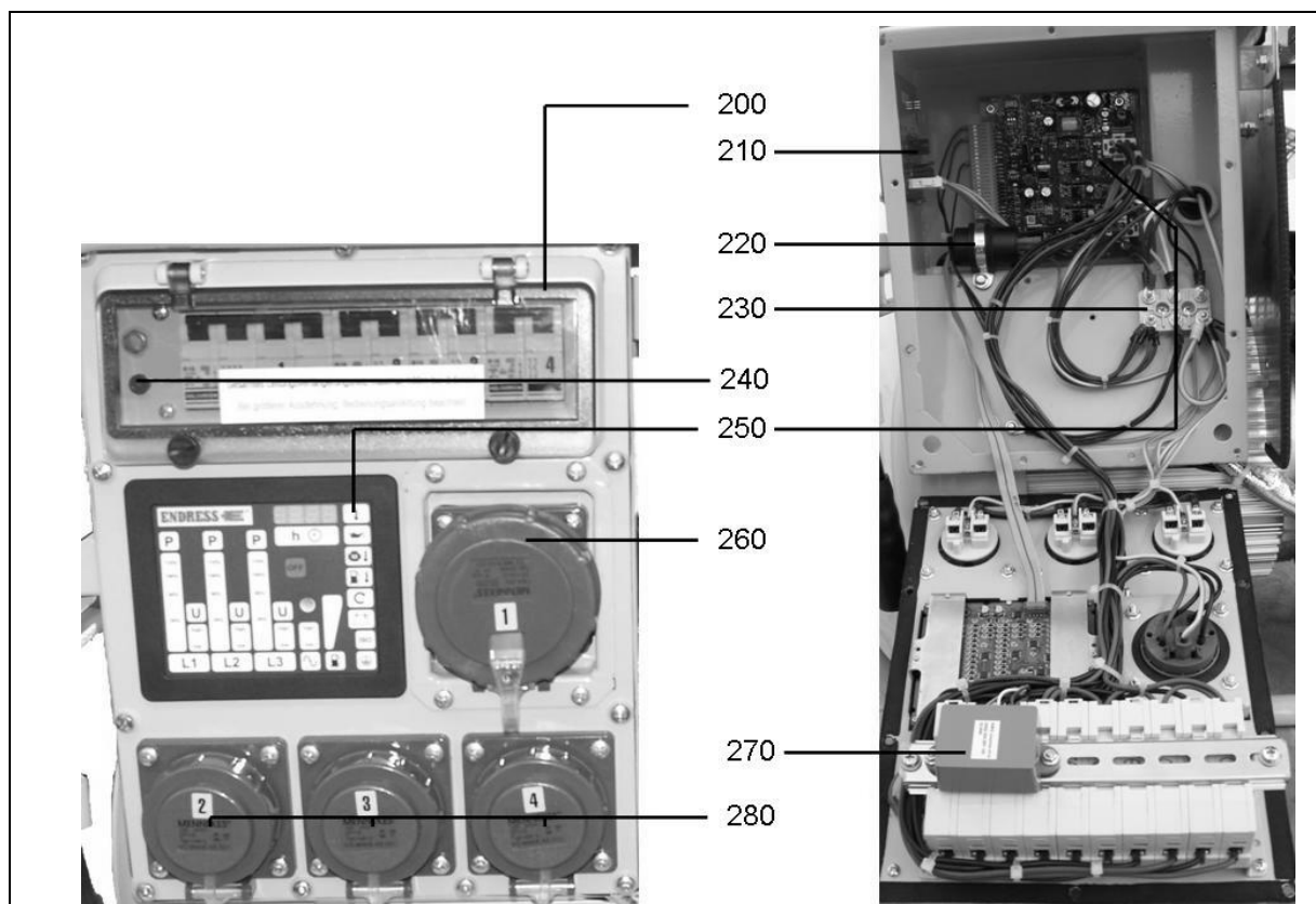
Abb. 9-3: Ersatzteile Generator und Elektronik
