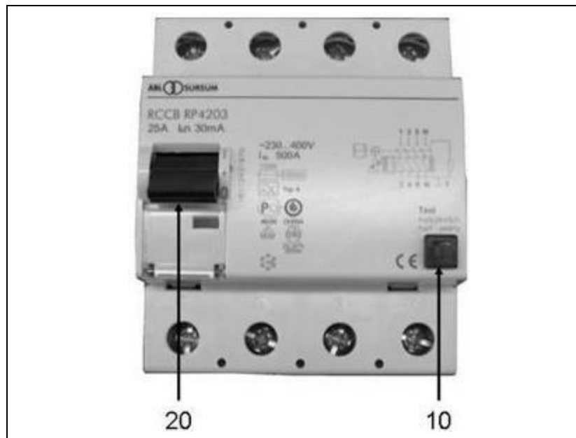
Abb. 5-1: FI-Schutzschalter
