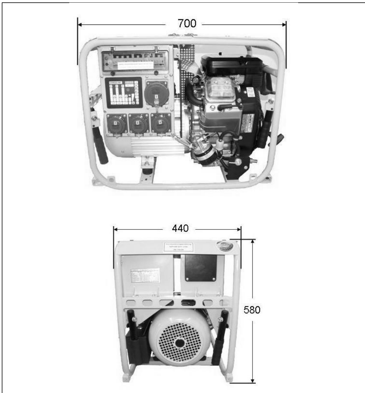
Abb. 8-1: Maße des Stromerzeugers
