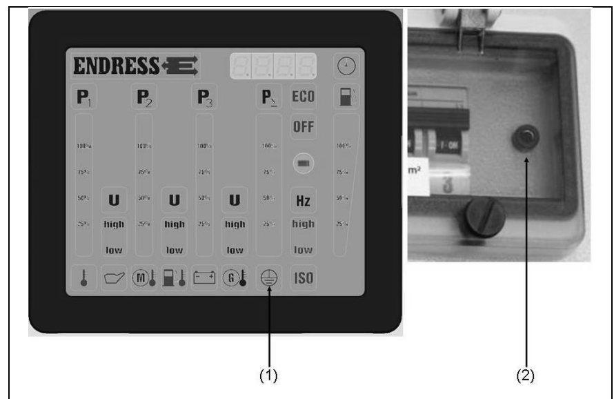
Abb. 4-4: Schutzleiter prüfen
