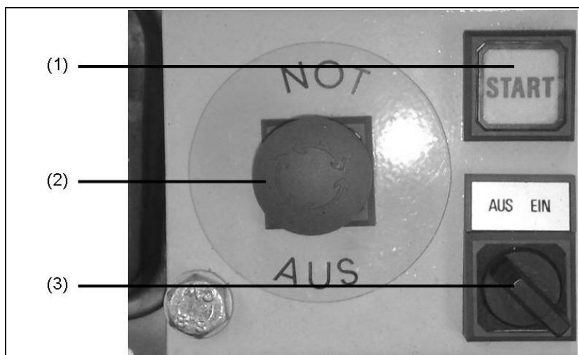
Abb. 5-5: Elektrostart in Verbindung mit Fernstart
