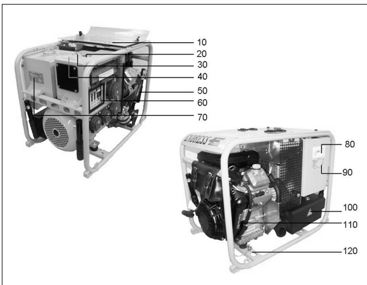
Abb. 2-1: Kennzeichnungen am Stromerzeuger
