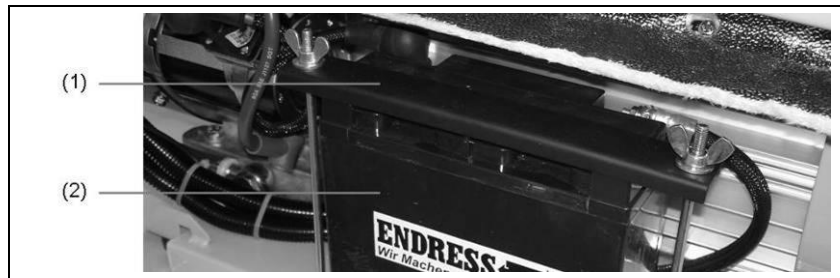
Abb. 6-3: Batterie wechseln
