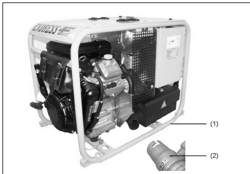
Abb. 5-13 Abgasschlauch anschließen
