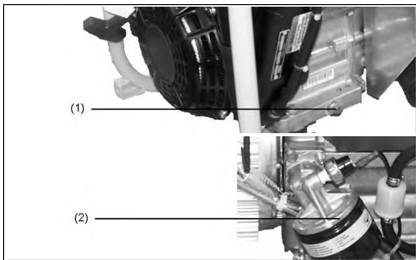
Abb. 6-2: Öl wechseln
