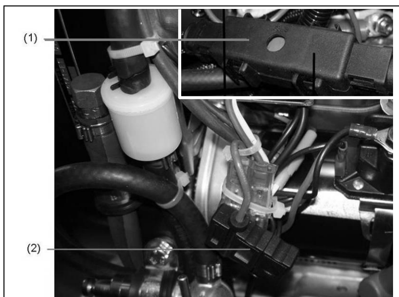
Abb. 6-4: Sicherung tauschen
