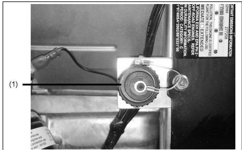
Abb. 5-4: Fernstarteinrichtung anschließen
