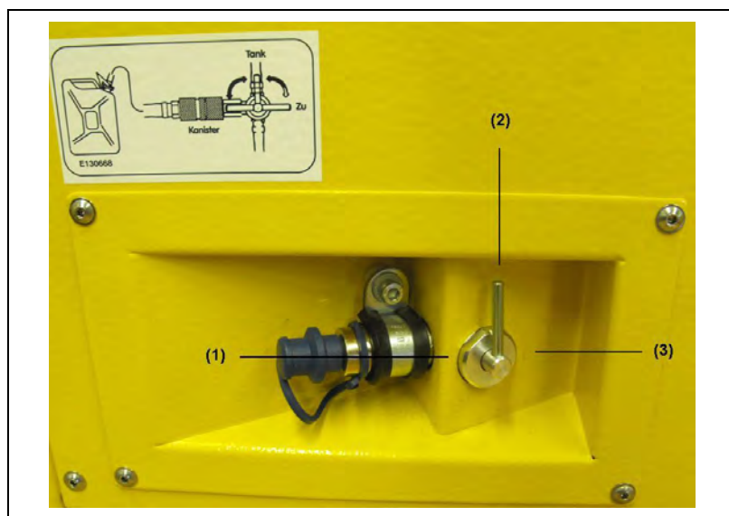
Abb. 5-11: 3 Wege Kraftstoffhahn
