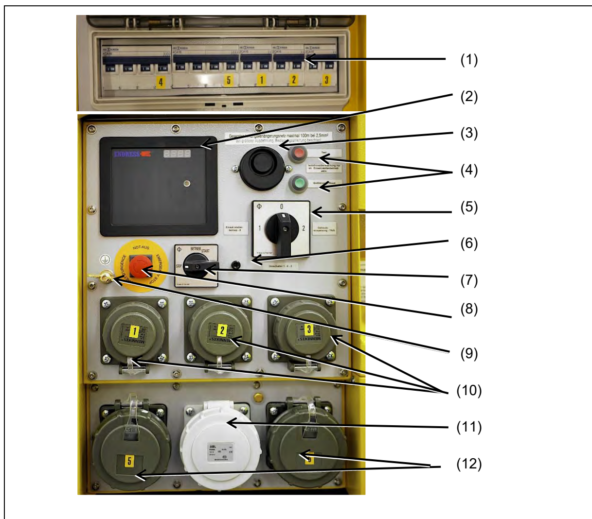
Abb. 3-4: Bestandteile des Elektrokastens
