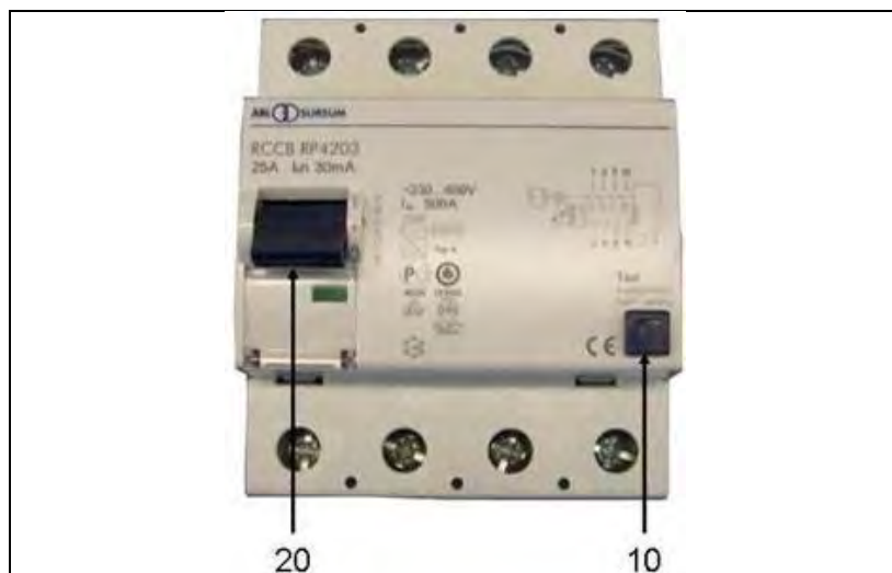
Abb. 5-1: FI-Schutzschalter
