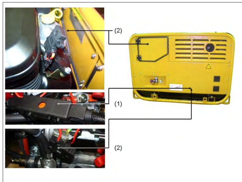
Abb. 6-4: Sicherung tauschen
