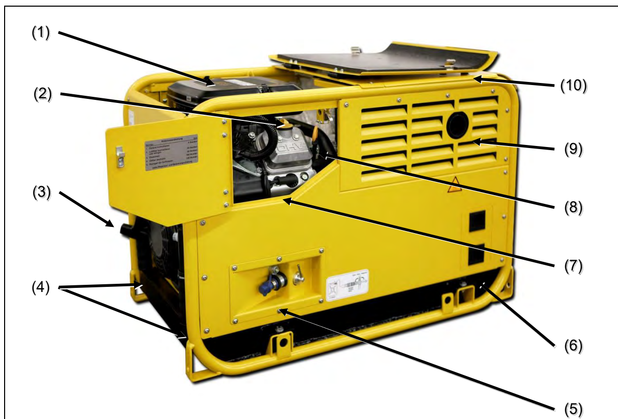
Abb. 3-3: Bestandteile der Abgas- und Generatorseite (Abbildung des Grundtyps)
