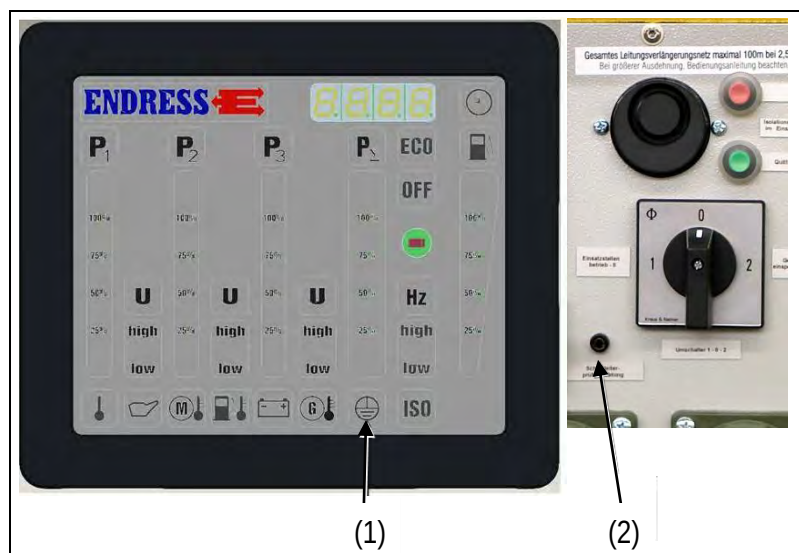
Abb. 4-4: Schutzleiter prüfen
