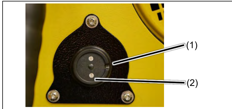
Abb. 5-9: MagCode Ladestrom-Steckdose
