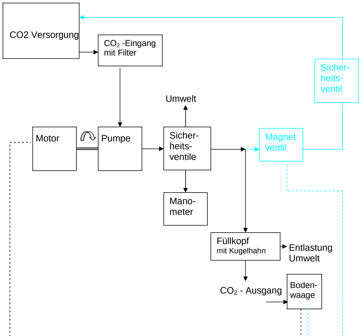
Blockschaltbild 4pro
