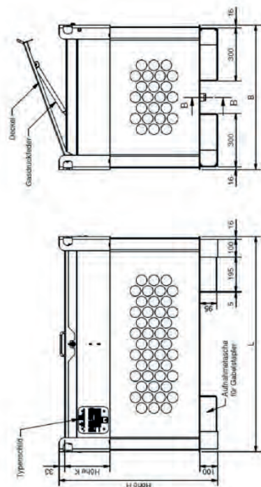
Übersichtszeichnung Typ "KC Quadro C..."
