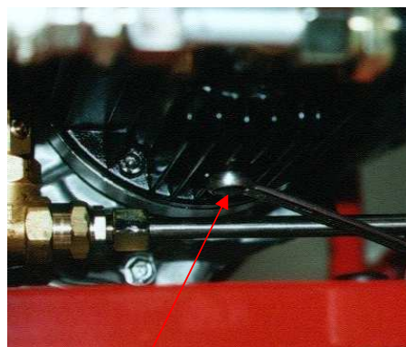
Pumpenölablassschraube
