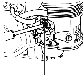
DROSSELANSCHLAGSCHRAUBE
