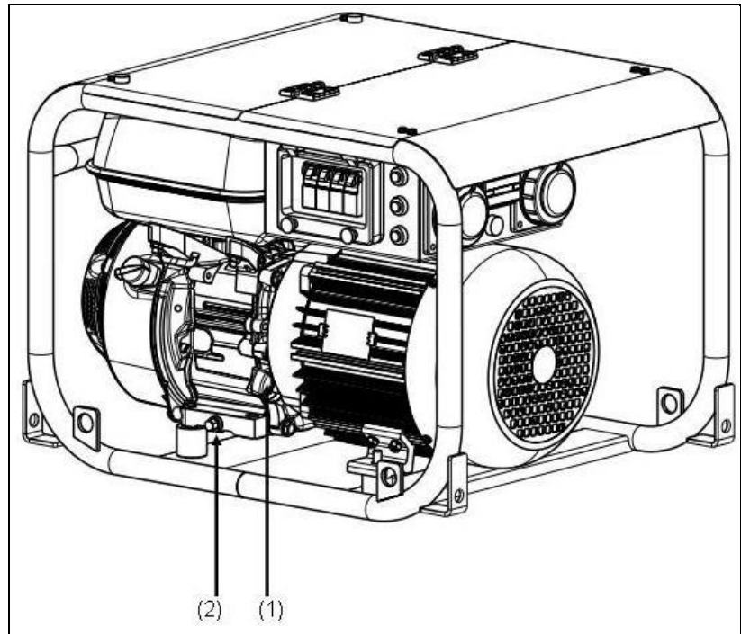
Abb. 6-1: Ölmesstab
