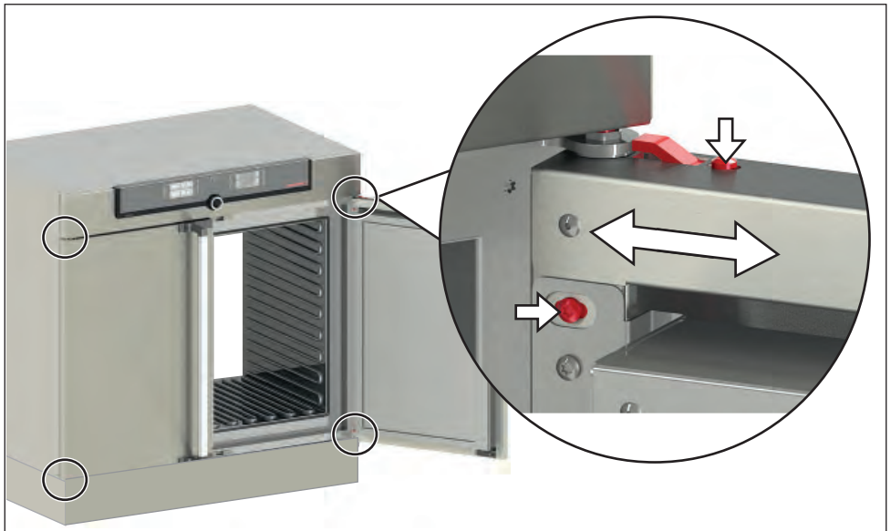
Abb. 12 Türeinjustierschrauben
