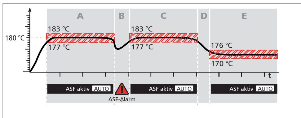
Abb. 23 Schematische Darstellung Funktionsweise ASF-Temperaturüberwachung
