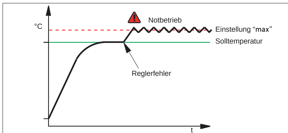
Abb. 21 Schematische Darstellung Funktionsweise TWW-Temperaturüberwachung
