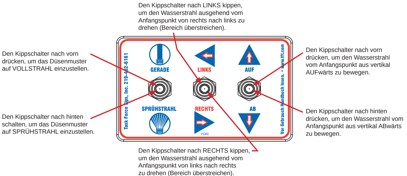
Abbildung 2.6.3 Aufkleber Bedienstation
