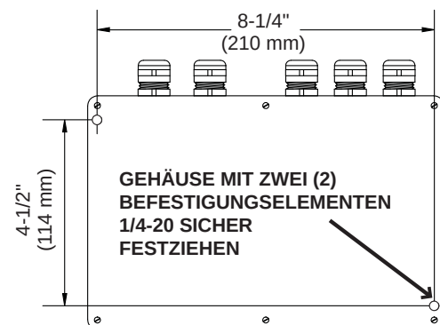
Abb. 2.10.1 Anordnung der Befestigungslöcher zur Elektrikgehäusemontage
