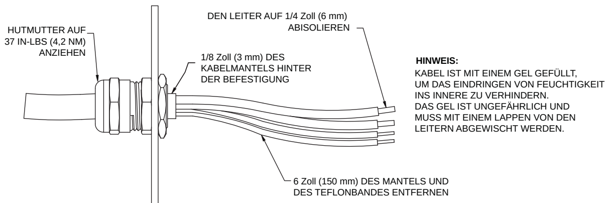
Abb. 2.2.2 Typische Kabelverlegung
