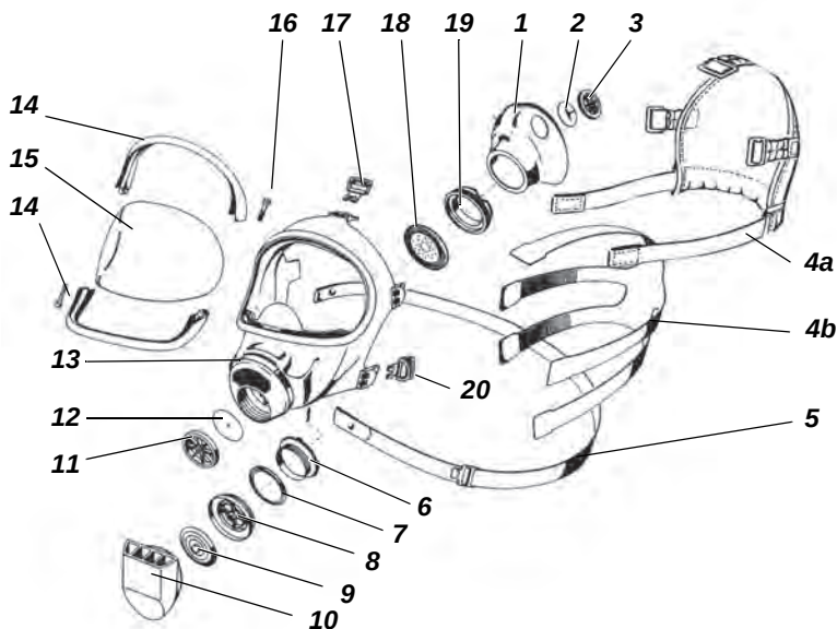
Abb. 3 Vollmaske, Explosionsdarstellung
