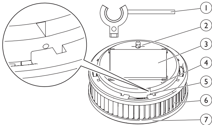
Abb. 1 Bedienelemente
