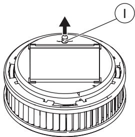
Abb. 9 Aktivierungstaste herausziehen
