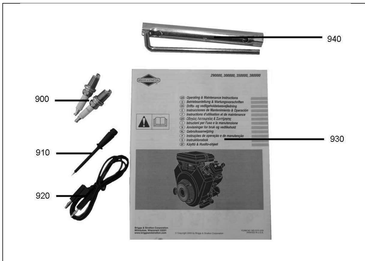
Abb. 9-6: Ersatzteile-Zubehör
