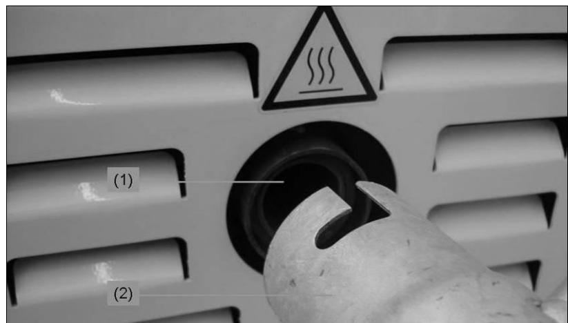
Abb. 5-13 Abgasschlauch anschließen
