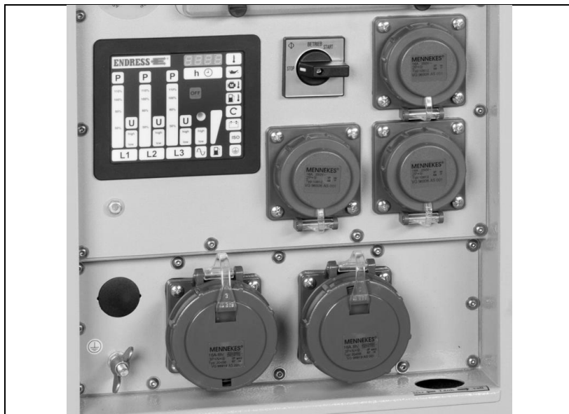
Abb. 4-5: Verbraucher anschließen
