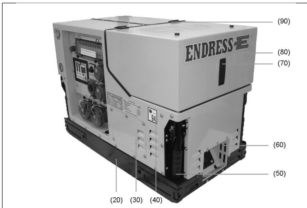
Abb. 9-1: Schalldämmhaube
