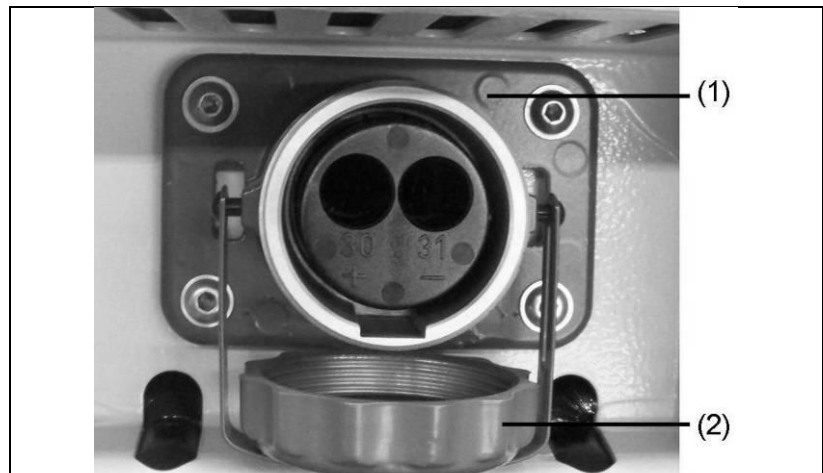
Abb. 5-6: Fremdstarteinrichtung anschließen
