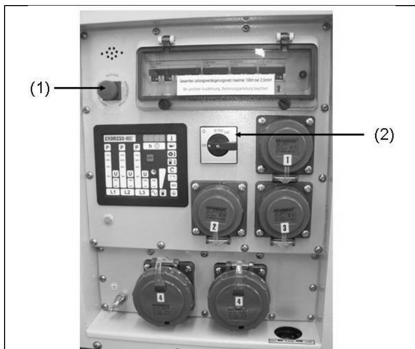
Abb. 4-2: Bedienpaneel Standardausführung
