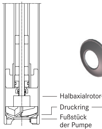
F/FP 430 mit Gleitringdichtung und Halbaxialrotor (Z-Version)
