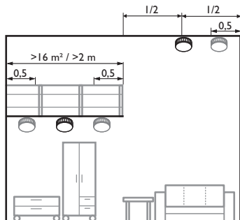
Abb. 9 Räume mit Podest oder Galerie
