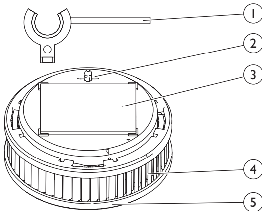
Abb. 3 Bedienelemente
