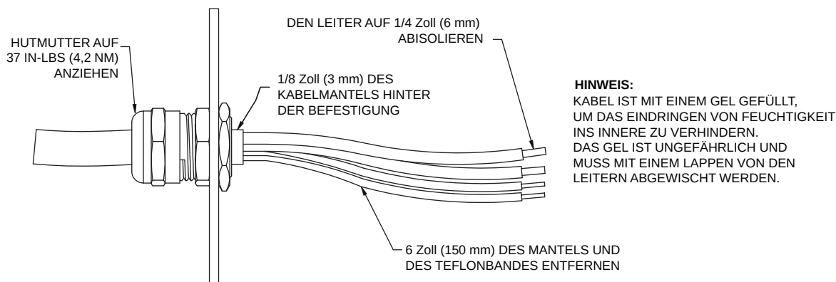
Abb. 2.2.2 Typische Kabelverlegung
