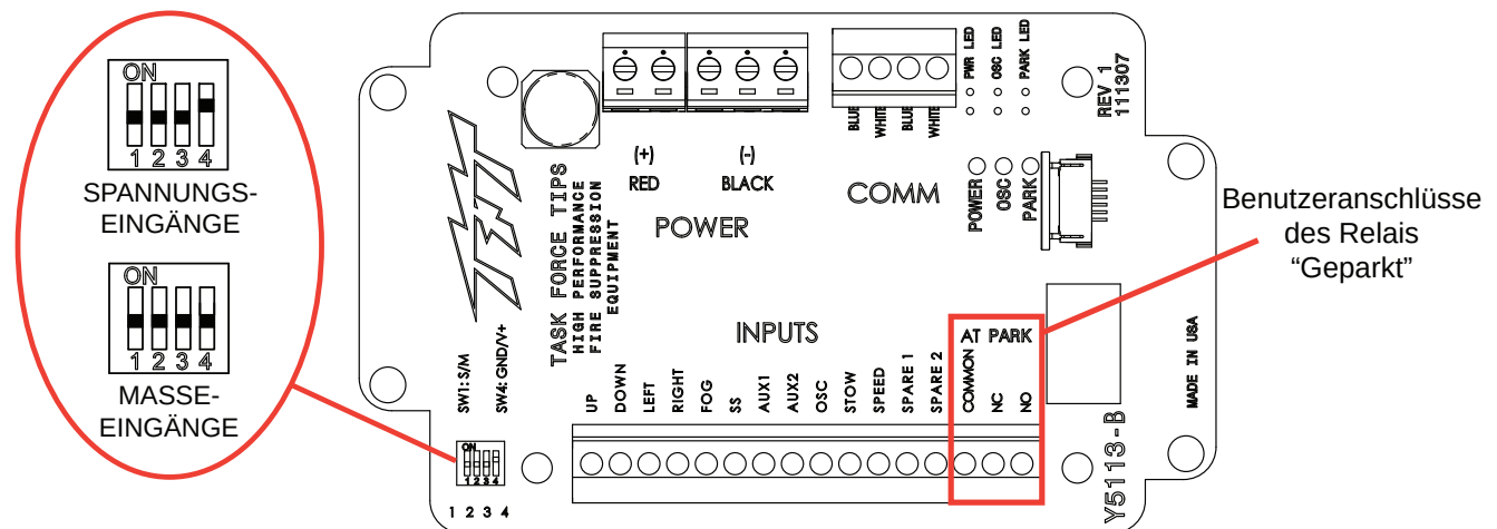
Abb. 2.7.3 Relais- und Anschlusslokalisierung
