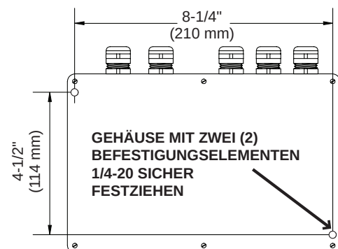
Abb. 2.10.1 Anordnung der Befestigungslöcher zur Elektrikgehäusemontage
