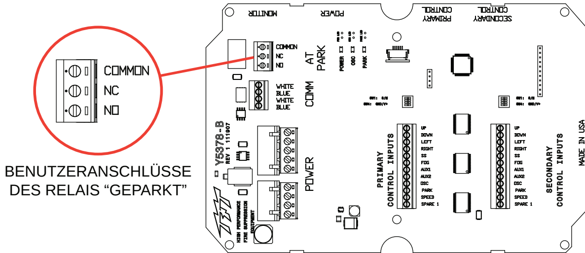
Abbildung 2.10.3.1 Relais und Anschlüsse
