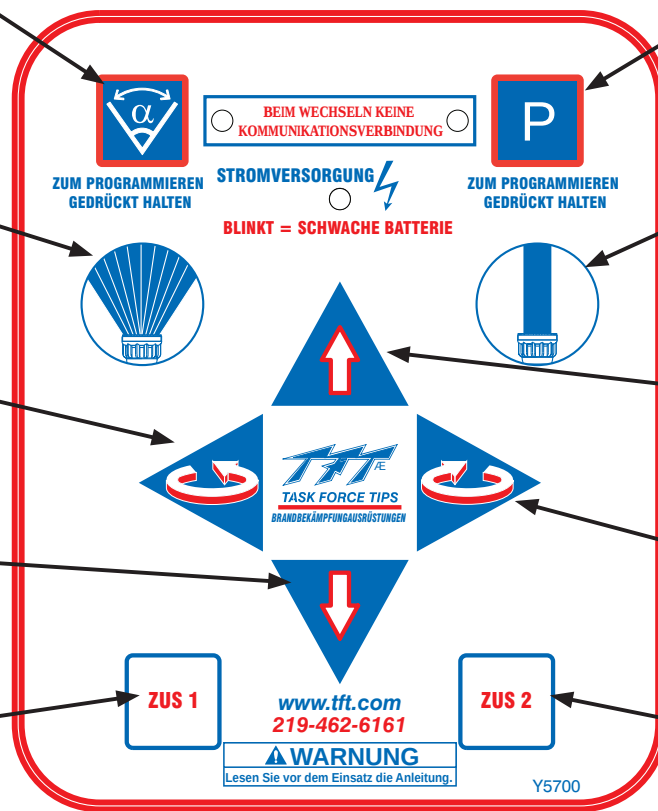
Abb. 2.2.5 Aufkleber Bedienung
