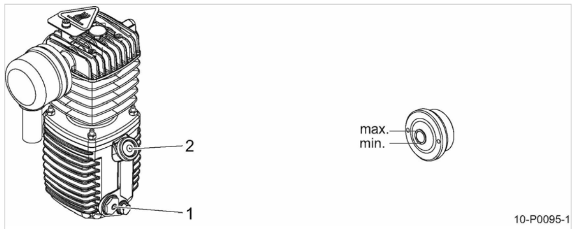
Abb. 10 Kompressorölstand prüfen
