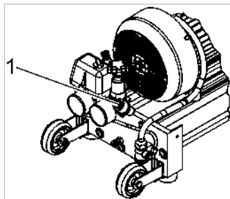
Abb. 3 Druckluftanschluss
