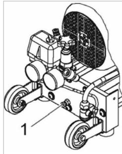
Abb. 15 Maschine entlüften
