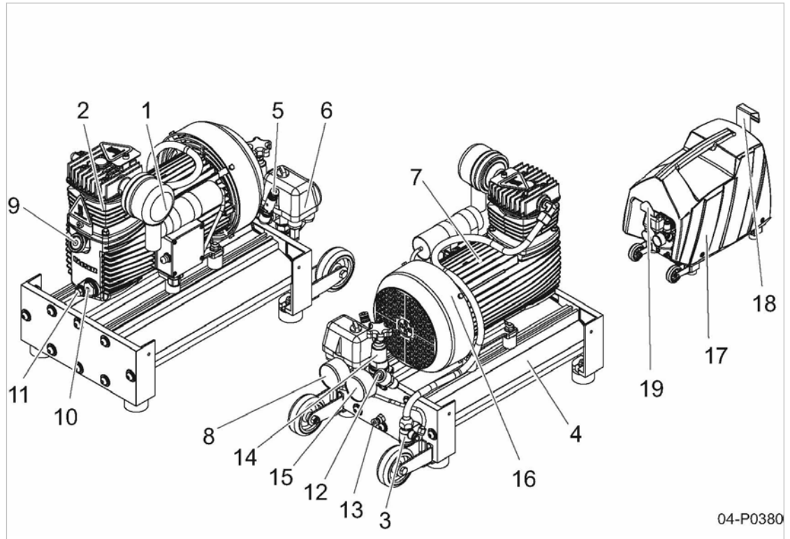
Abb. 2 Übersicht Maschine
