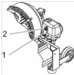
Abb. 13 Sicherheitsventil am Druckluftbehälter prüfen
