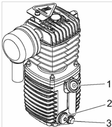
Abb. 12 Kompressoröl wechseln
