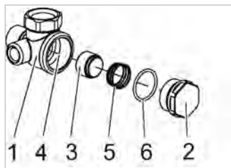
Abb. 16 Rückschlagventil reinigen
