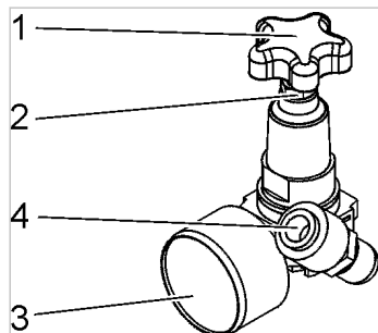
Abb. 6 Druckminderer einstellen
