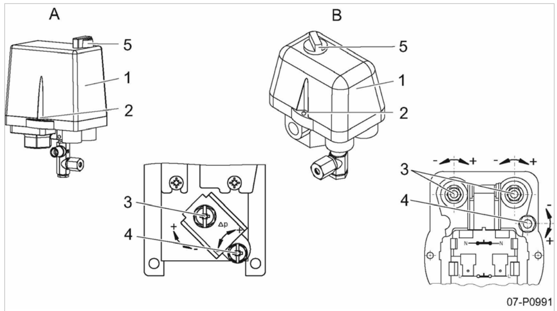
Abb. 5 Netzdruck einstellen
