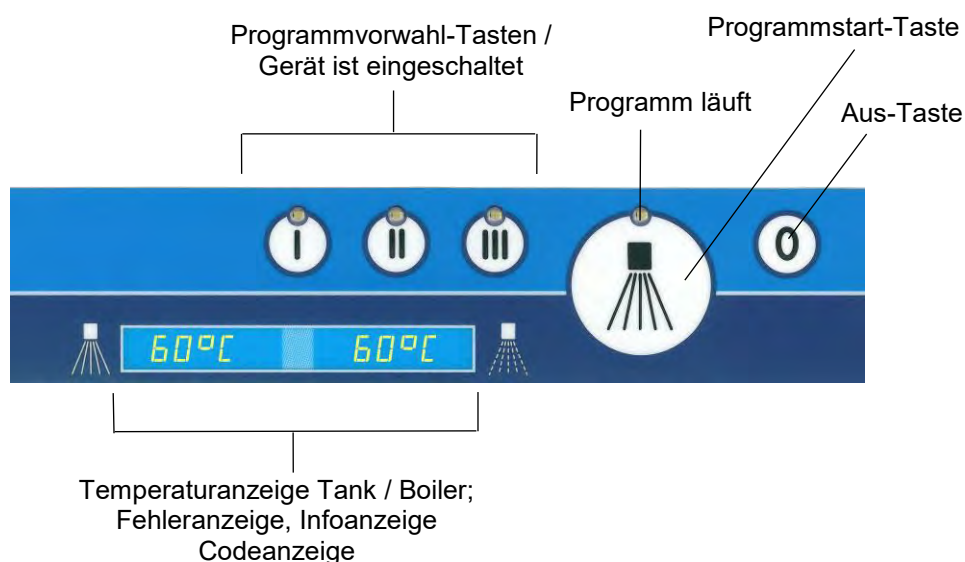
Abbildung 1; Bedientastatur
