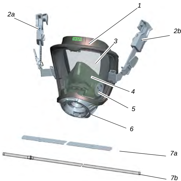
Abb. 1 Übersicht Masken-Helm-Kombination
