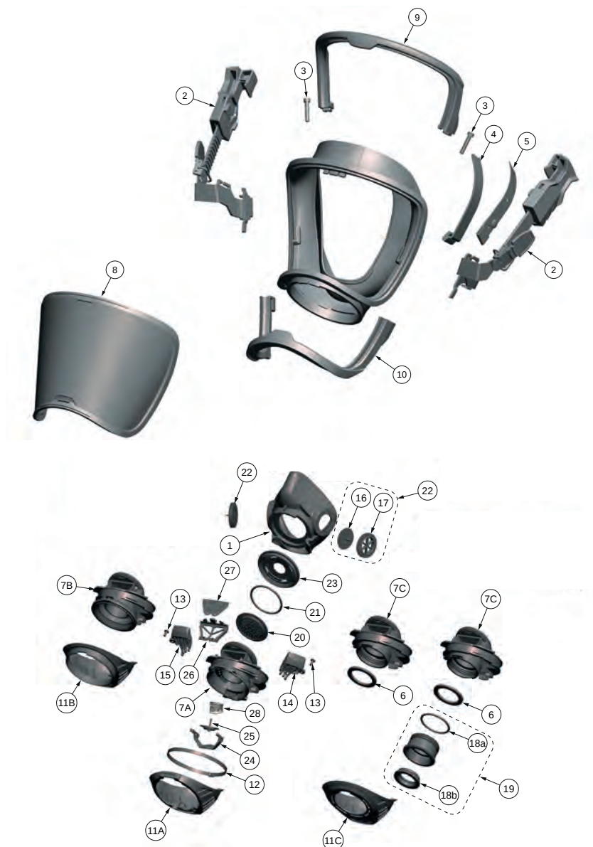
Abb. 8 G1-H-Maske – Überdruck
