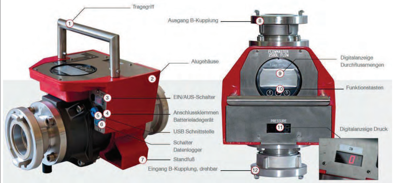
Abb. 3.2: Beschreibung der Hauptkomponenten des digitalen Flowmasters Typ 250DL
