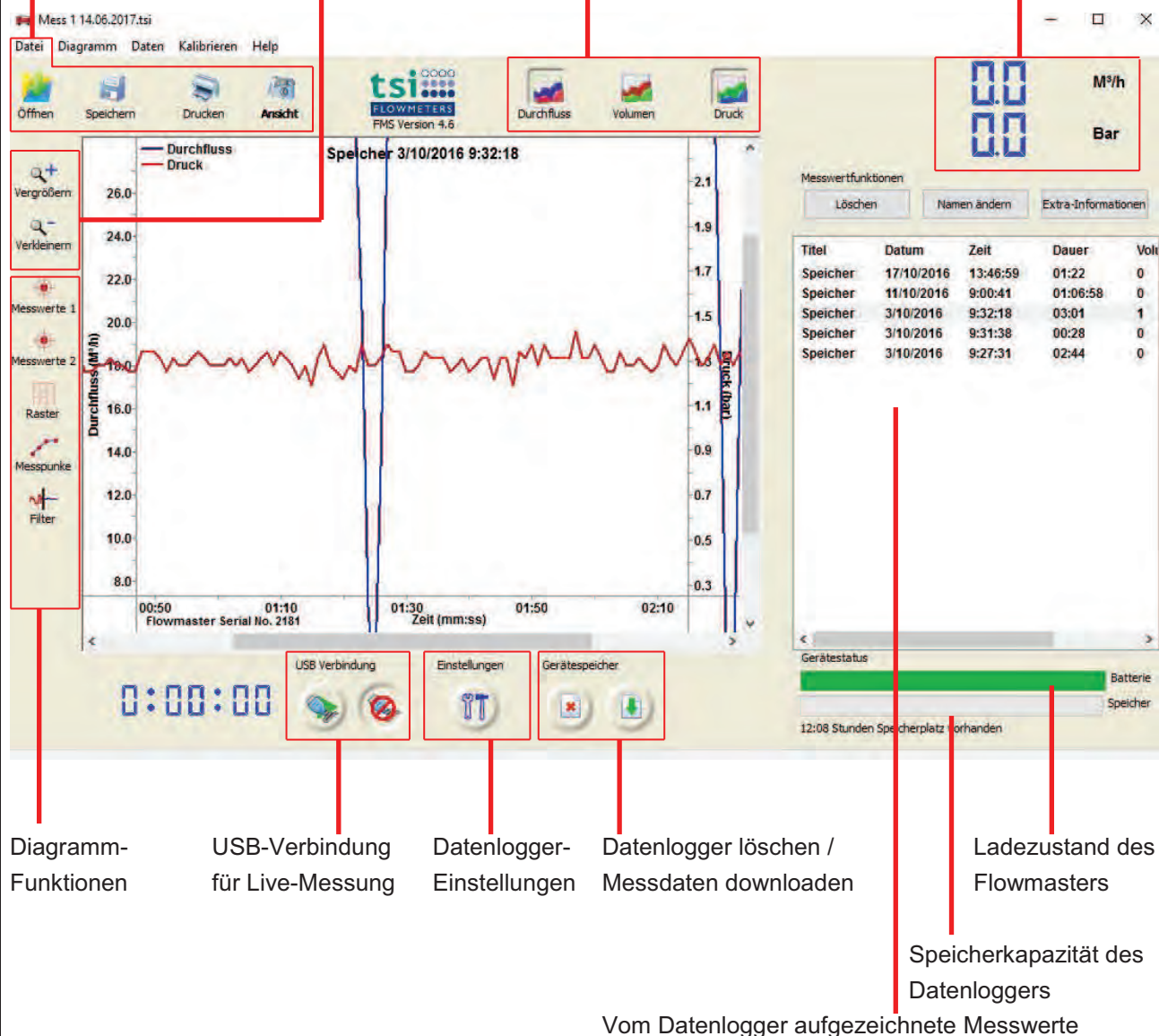
Abb. 5.2: Desktopbild der Flowmaster-Software Version 4.6
