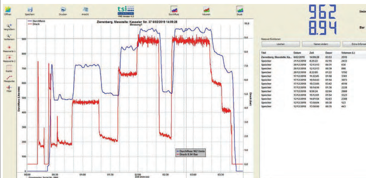
Abb. 5.8: Messwert-Diagramm anpassen
