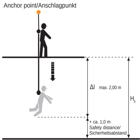
Abb. 6 Definition of the required ground clearance/ Bestimmung des benötigten Bodenfreiraums
