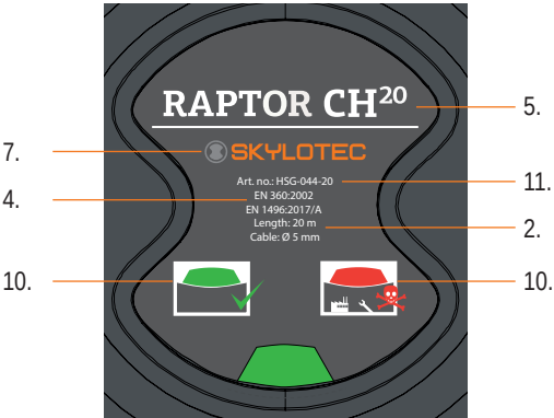
Abb. 6 rear view - RAPTOR CH20 (with lifting function)/ Rückseite - RAPTOR CH20 (mit Hubfunktion)
