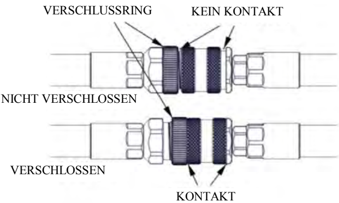
Abbildung 2-1 Schnellkupplungs-Sicherheitsverschlussring
