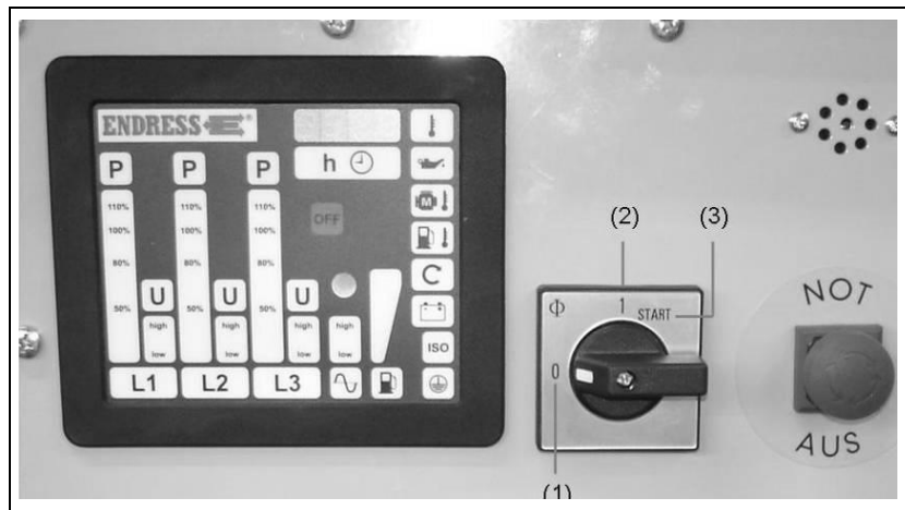
Abb. 4-2: Bedienpanel Standardausführung
