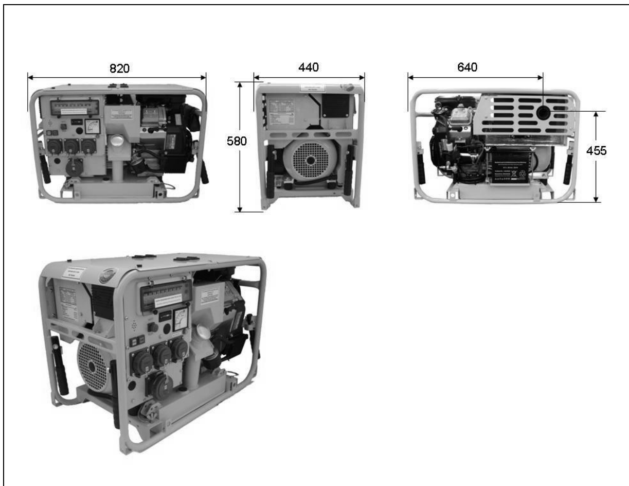
Abb. 8-1: Maße des Stromerzeugers
