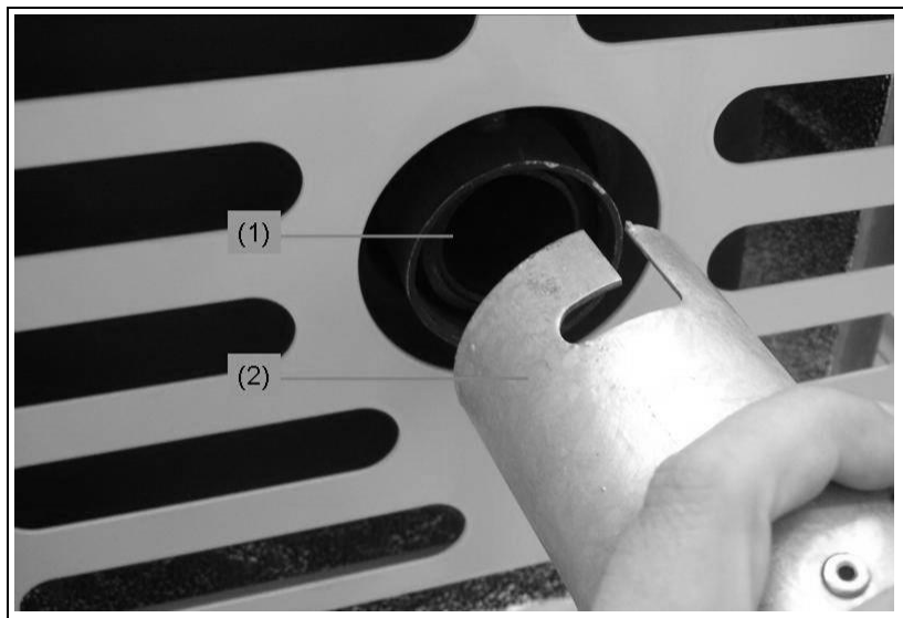
Abb. 5-13 Abgasschlauch anschließen
