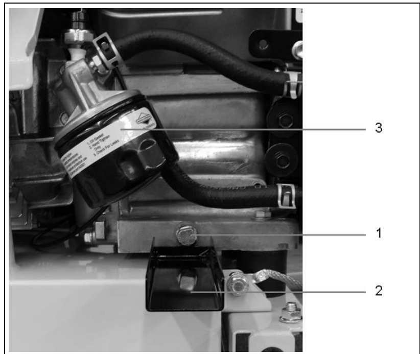
Abb. 6-3: Öl wechseln
