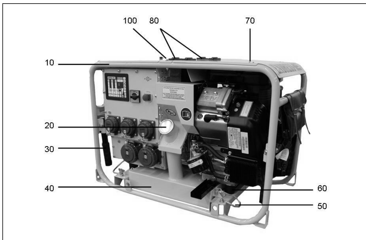
Abb. 9-1: Ersatzteile der Bedien- und Generatorseite
