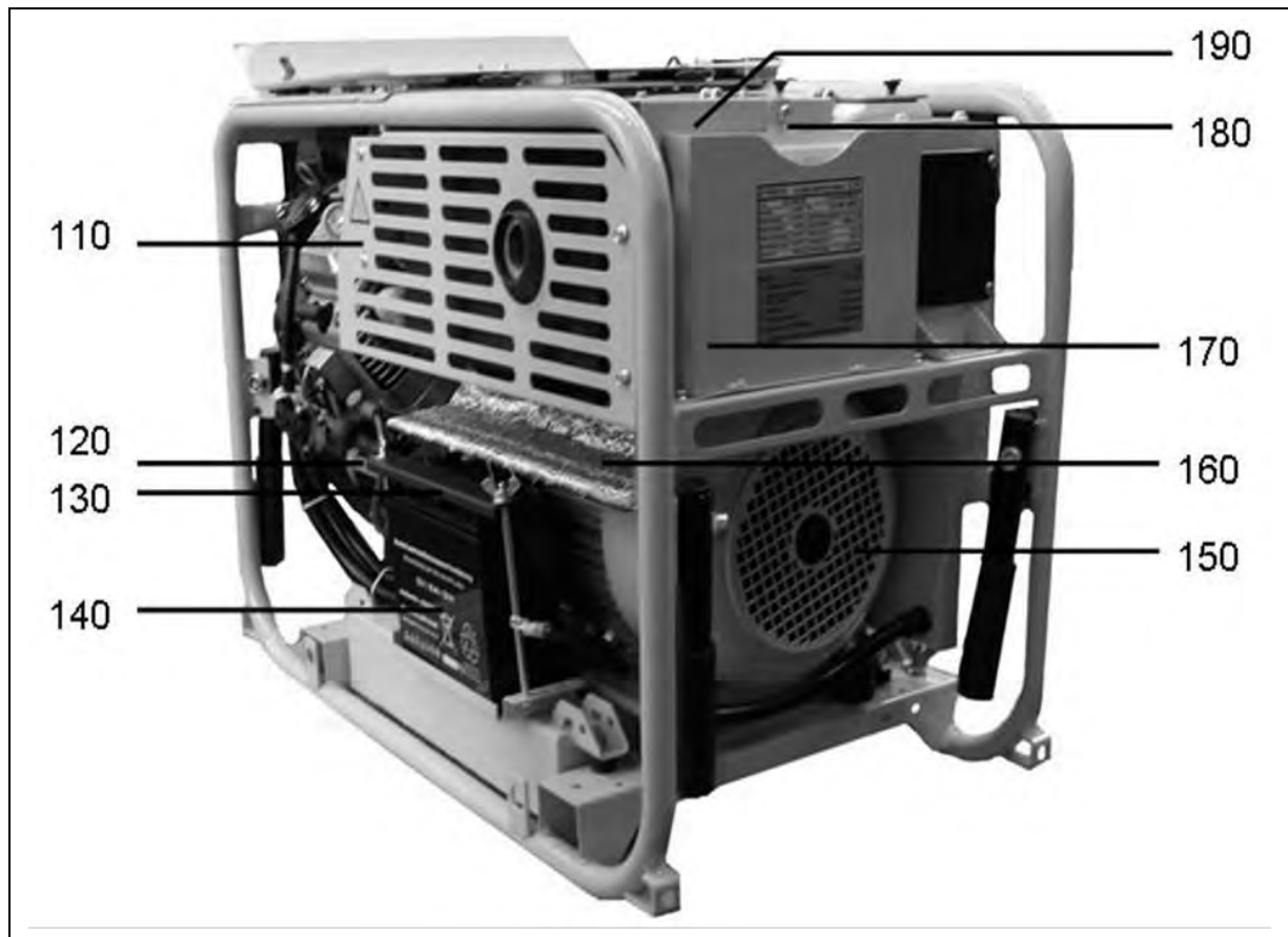
Abb. 9-2: Ersatzteile der Motor- und Abgasseite
