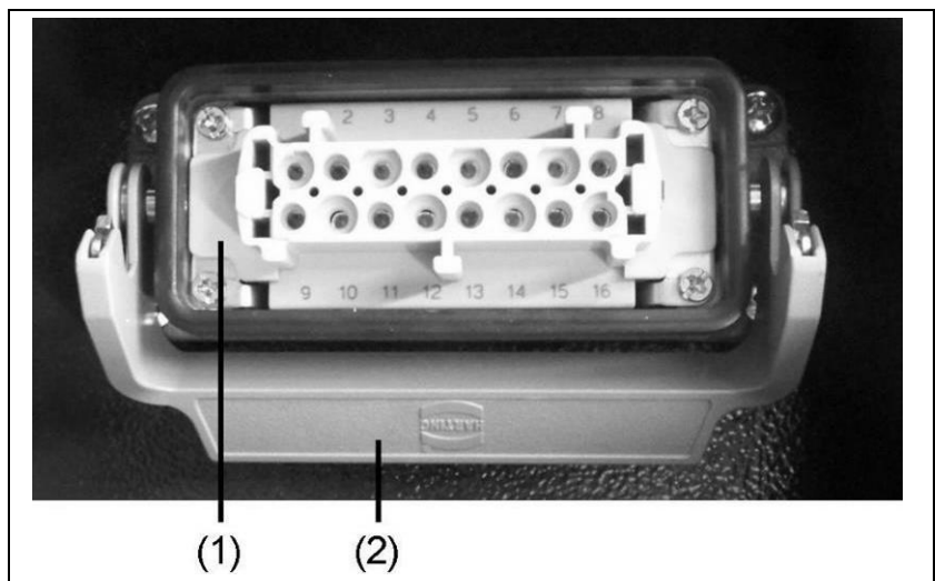
Abb. 5-4: Fernstarteinrichtung mit Harting-Stecker
