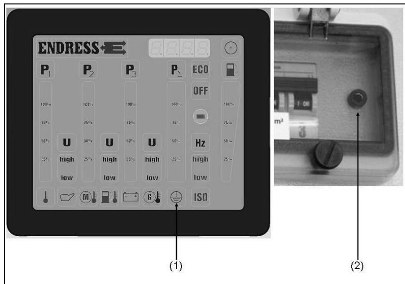
Abb. 4-5: Schutzleiter prüfen
