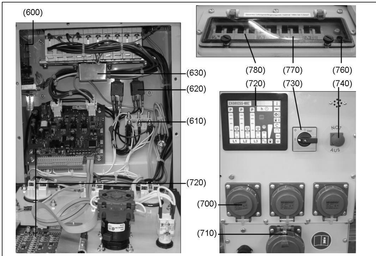
Abb. 9-4: Ersatzteile Generator und Elektronik
