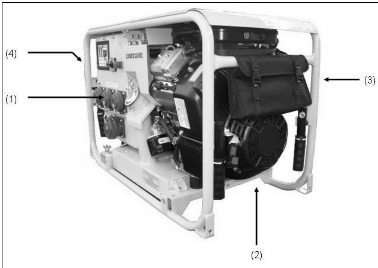
Abb. 3-1: Ansichten des Stromerzeugers
