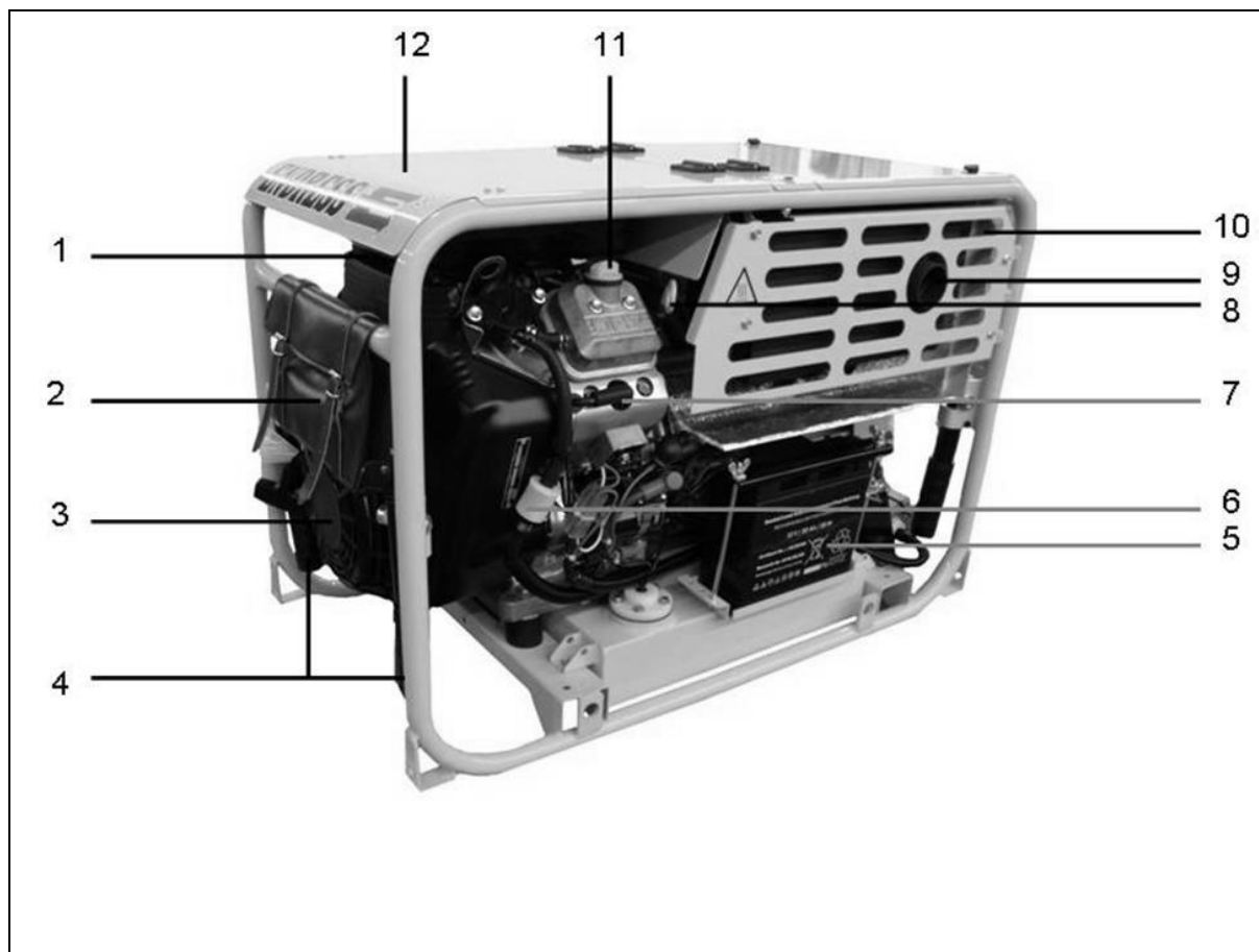
Abb. 3-3: Bestandteile der Abgas- und Motorseite
