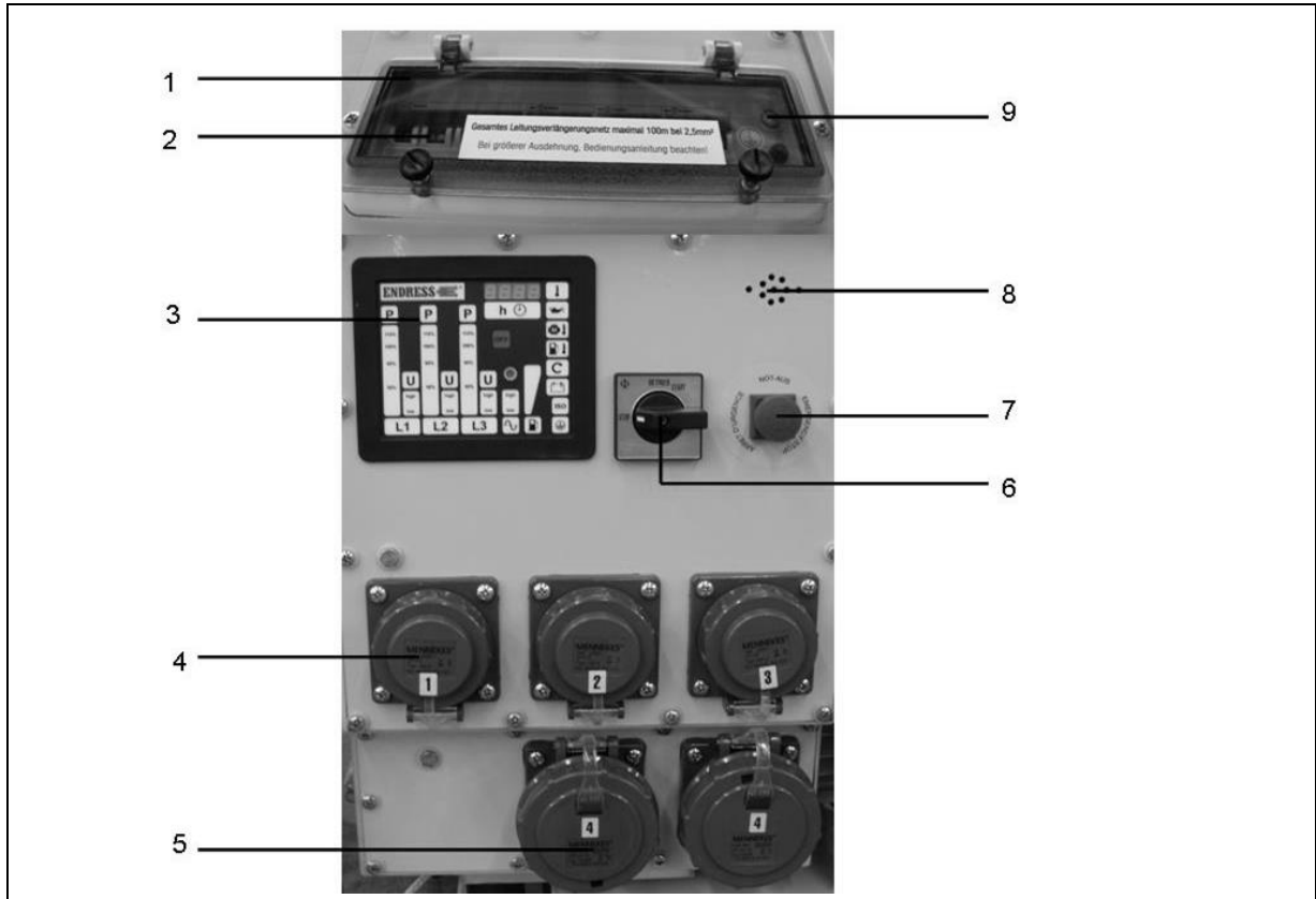
Abb. 3-4: Bestandteile des Elektrokastens
