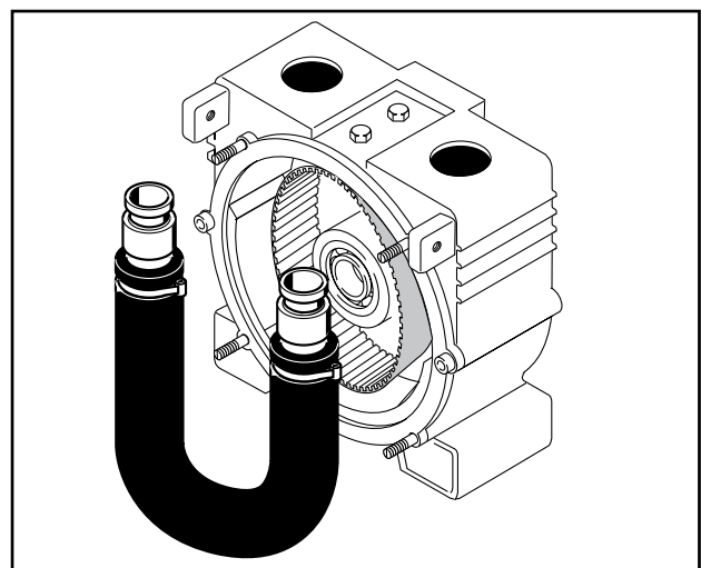
Abb. 19 Demontage Förderschlauch
