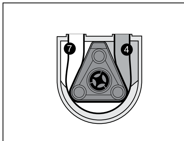
Abb. 6 4 Saugraum 7 Druckraum
