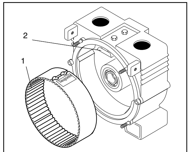
Abb. 20 Montage Trennteil
