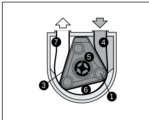
Abb. 5 1 Rotor 5 Innenraum 3 Trennteil 6 Schlauchkammer 4 Saugraum 7 Druckraum
