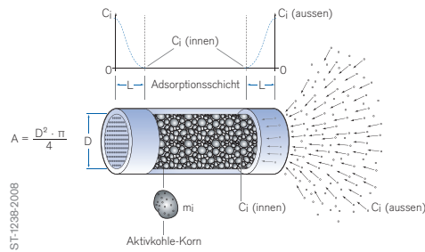
Messprinzip der passiven Probenahme mit dem Diffusionssammler ORSA.
