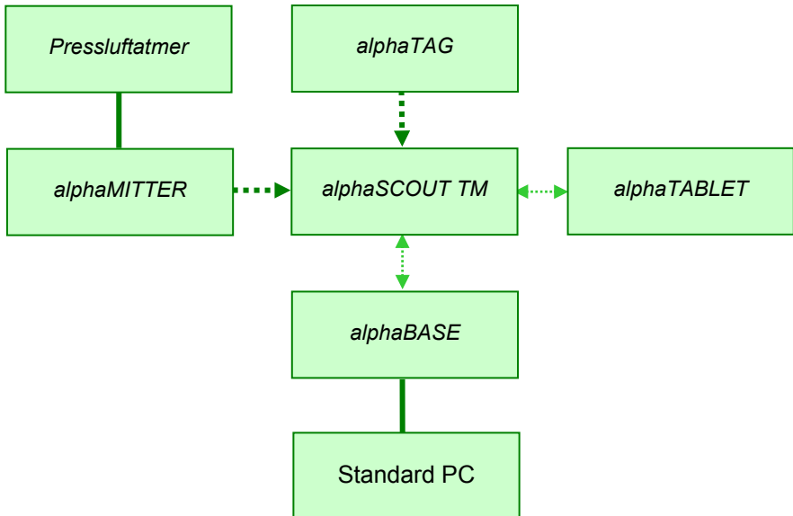
Bild 1 Systemübersicht
