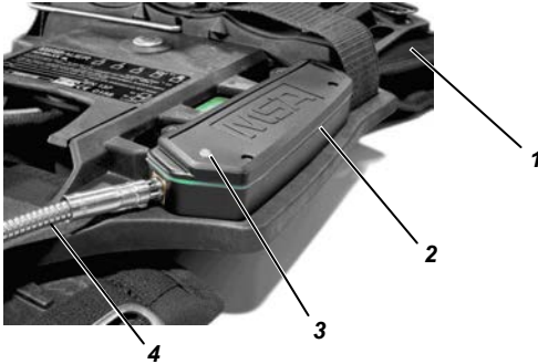
Bild 2 alphaMITTER
