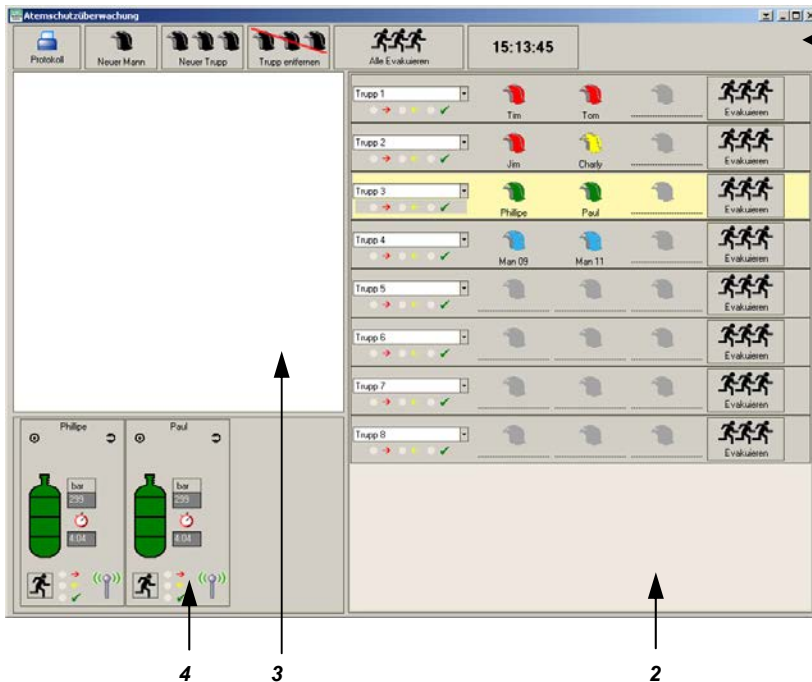
Bild 8 Benutzeroberfläche Telemetrie-Überwachungssoftware
