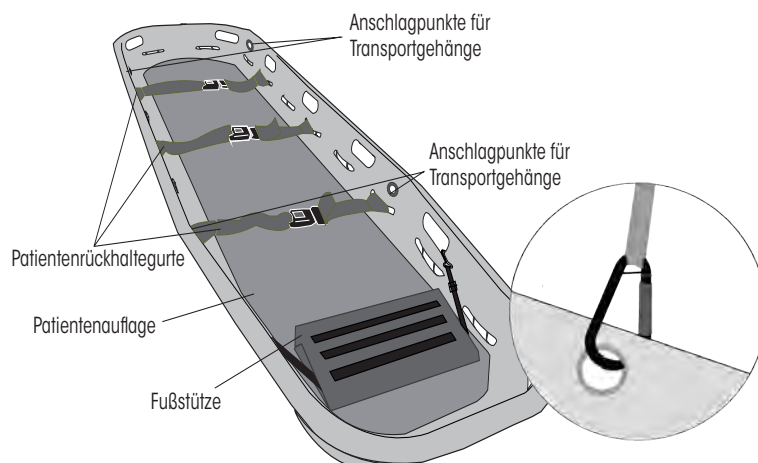
Bild 1: Teile der Korbtrage und Anschlagpunkte
