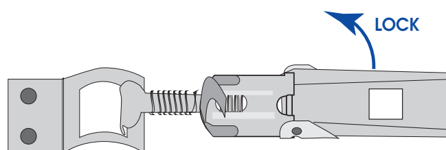
Bild 5: Verriegelung der äußeren Schnellverschlüsse
