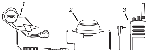
Abb. 13 Anschlussübersicht
