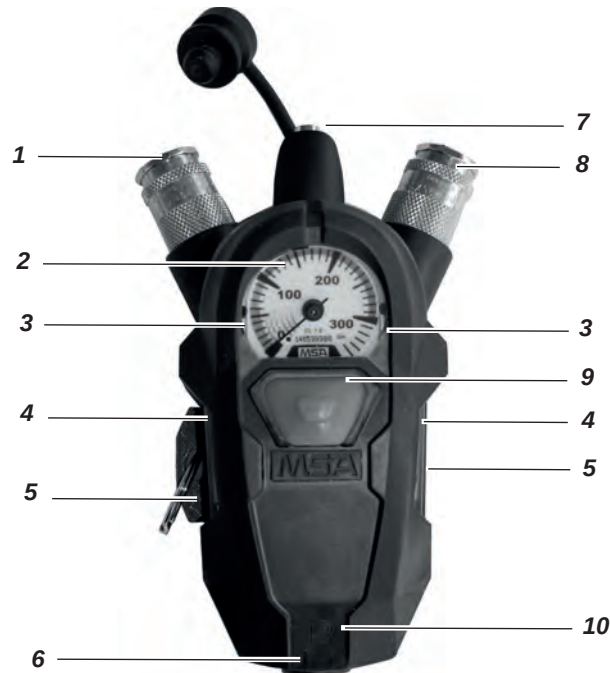
Abb. 1 Übersicht SingleLine SCOUT
