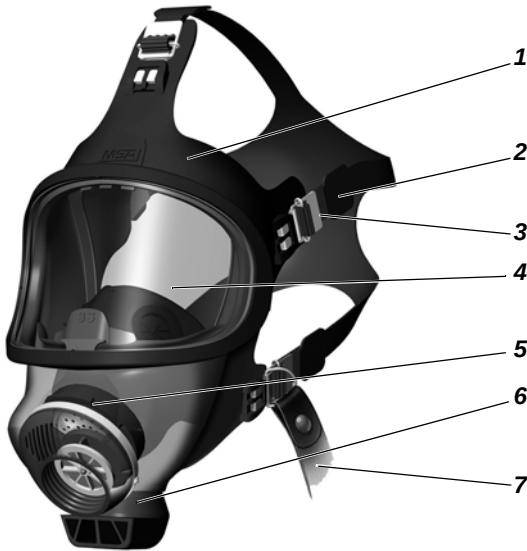
Abb. 1 Übersicht Vollmaske
