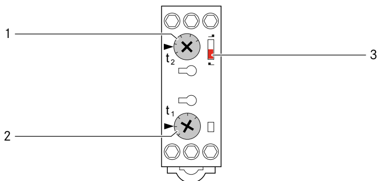
Abb. 35 Zeitrelais
