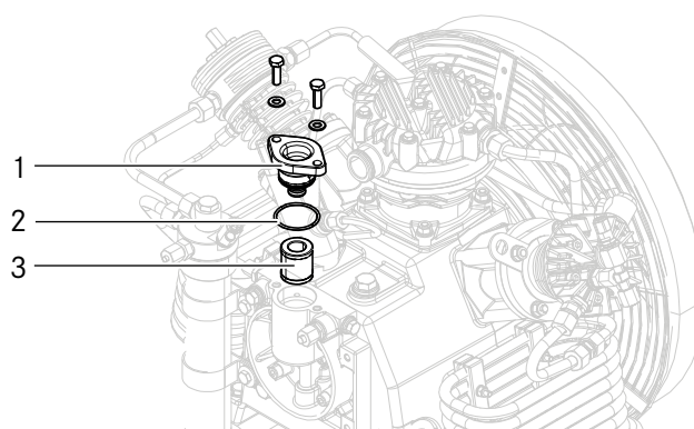
Abb. 24 Ölfilter tauschen
