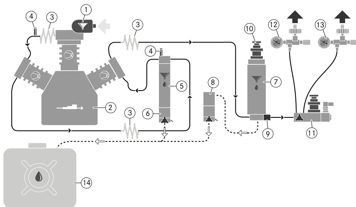
Abb. 6 Funktionsschema
