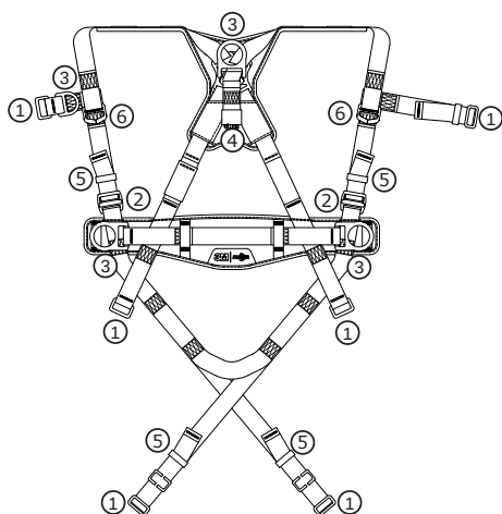
1. ábra – Fém tartozékok
