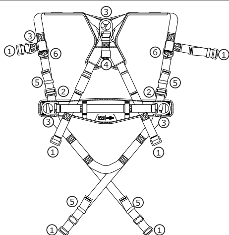
Диаграма 1 - Метални части
