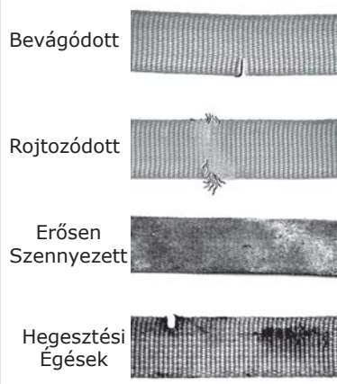
2. ábra – Heveder szövetek
