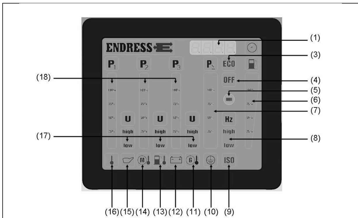
Abb. 4-7: Multifunktionsdisplay
