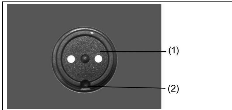
Abb. 5-9: MagCode Ladestrom-Steckdose
