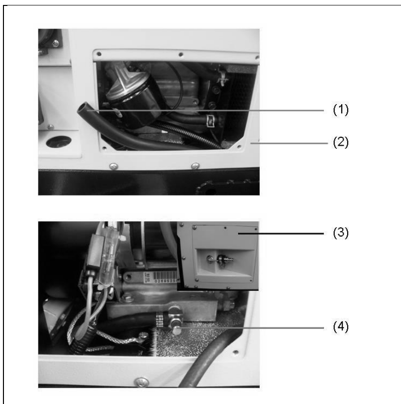
Abb. 6-3: Öl wechseln
